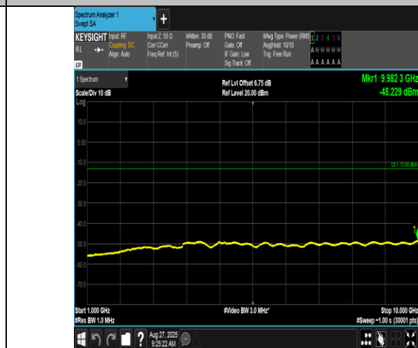
EGPRS850-251-8-1000~10000MHz-PASS
