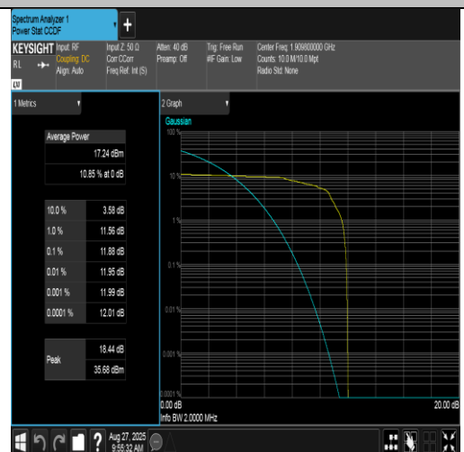
EGPRS1900-810-2-PASS
