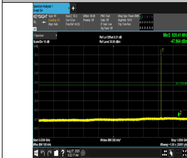
EGPRS850-128-8-30~1000MHz-PASS
