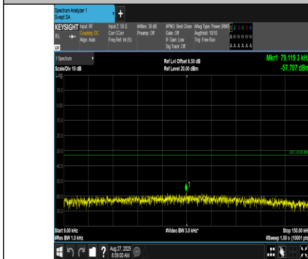
GPRS850-251-5-0.009~0.15MHz-PASS
