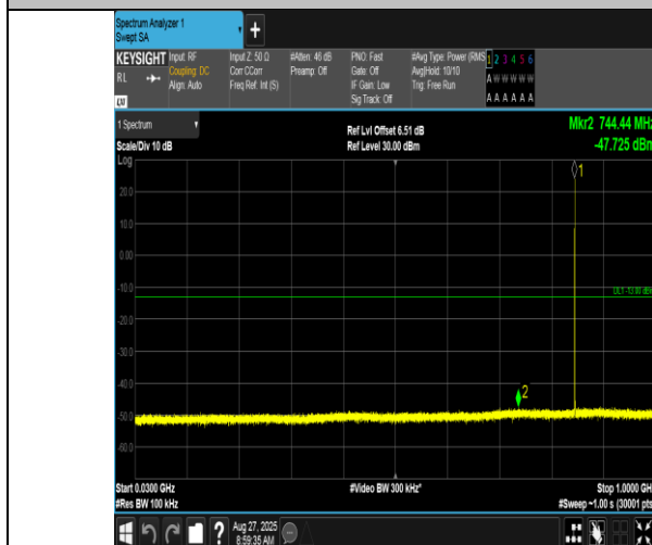
GPRS850-251-5-30~1000MHz-PASS
