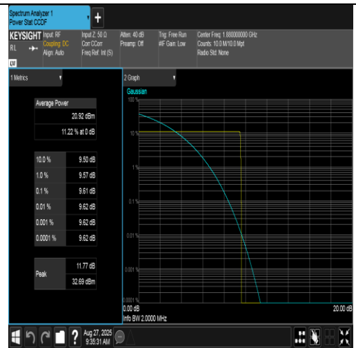
GPRS1900-661-0-PASS
