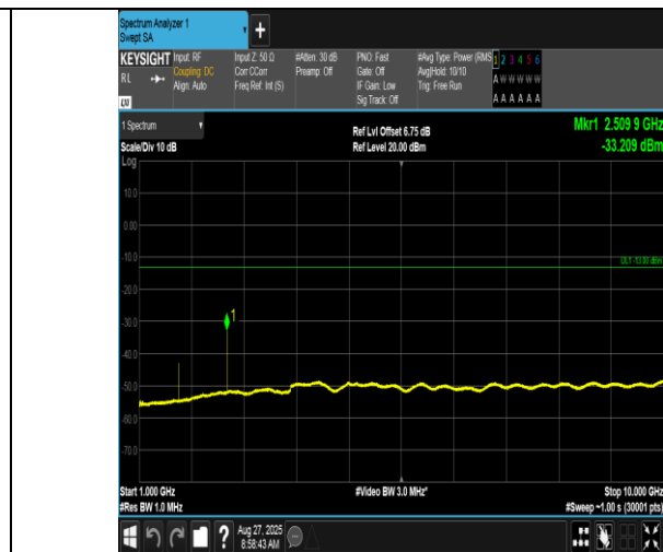
GPRS850-190-5-1000~10000MHz-PASS
