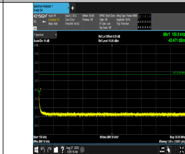
GPRS850-251-5-0.15~30MHz-PASS
