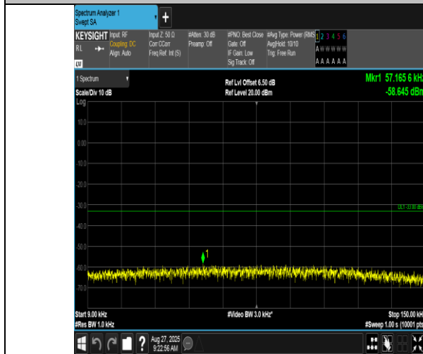
EGPRS850-190-8-0.009~0.15MHz-PASS
