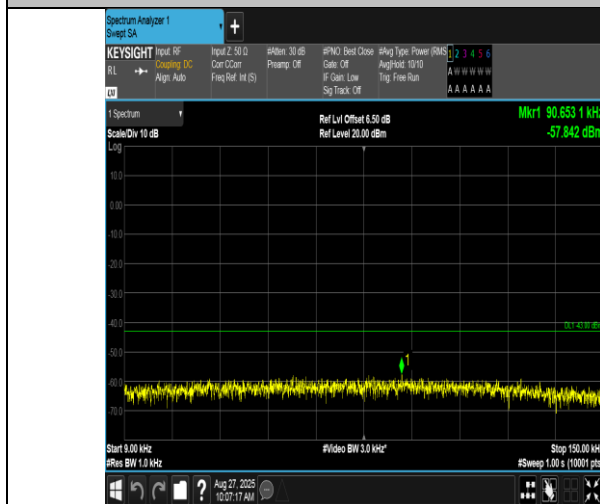
EGPRS1900-661-2-0.009~0.15MHz-PASS
