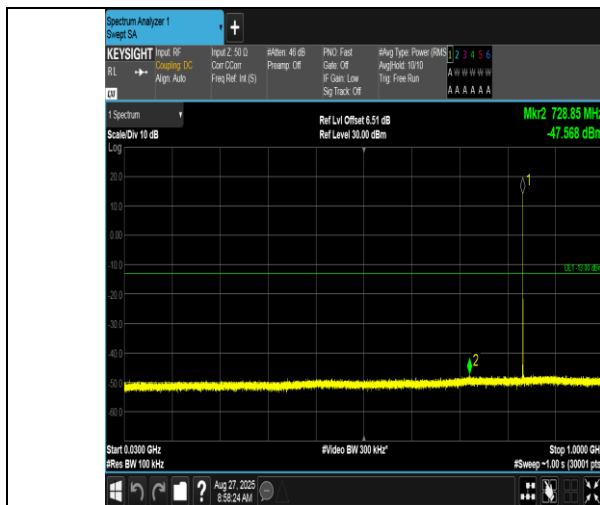
GPRS850-190-5-30~1000MHz-PASS
