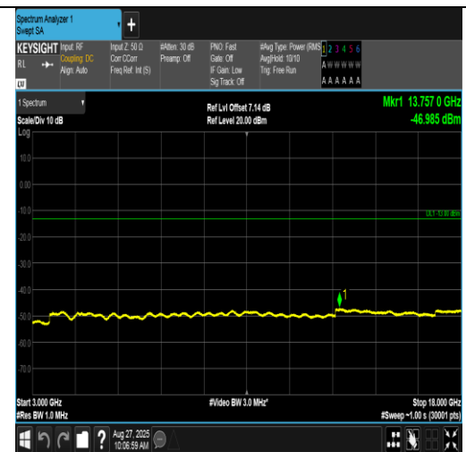
EGPRS1900-512-2-3000~18000MHz-PASS
