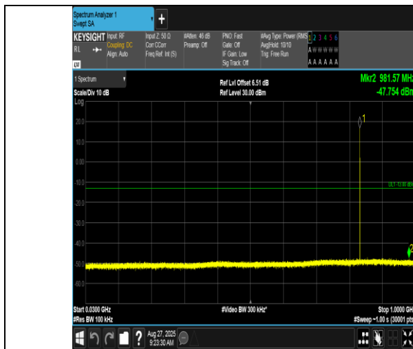
EGPRS850-190-8-30~1000MHz-PASS
