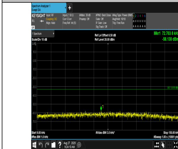
EGPRS850-251-8-0.009~0.15MHz-PASS
