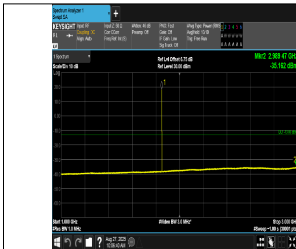
EGPRS1900-512-2-1000~3000MHz-PASS
