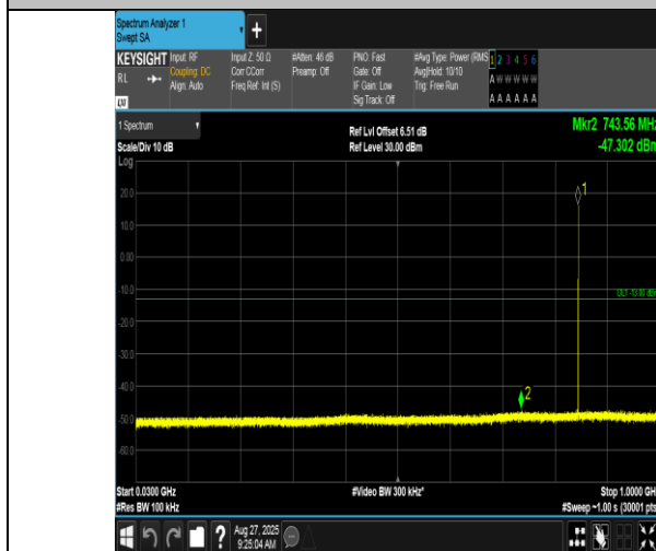
EGPRS850-251-8-30~1000MHz-PASS
