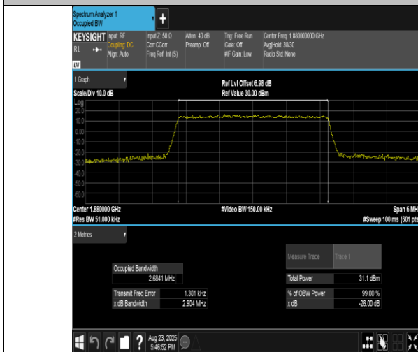
Band2-3MHz-QPSK-18900-15RB#0-PASS
