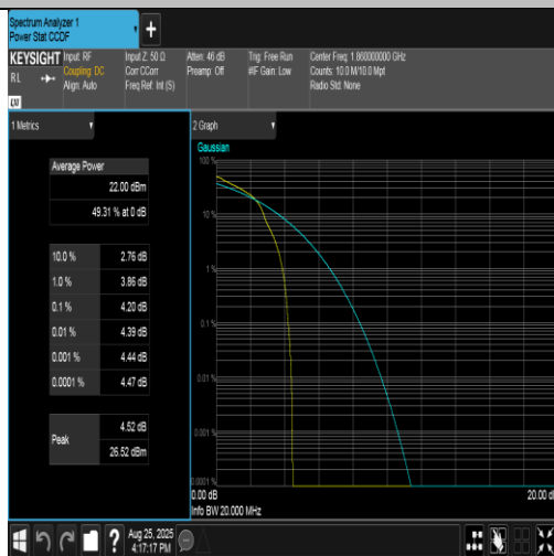
Band2-20MHz-16QAM-18700-1RB#0-PASS
