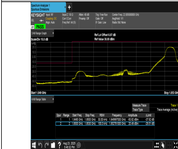
Band2-3MHz-16QAM-18615-1RB#14-PASS
