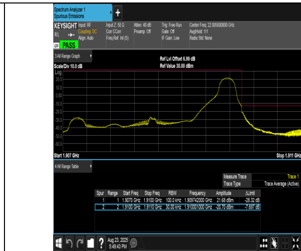
Band2-3MHz-QPSK-19185-1RB#14-PASS
