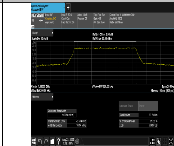
Band2-10MHz-16QAM-18900-50RB#0-PASS
