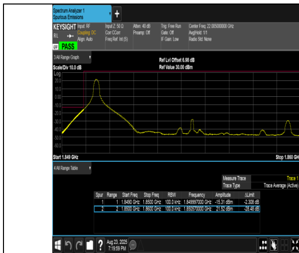
Band2-10MHz-QPSK-18650-1RB#0-PASS
