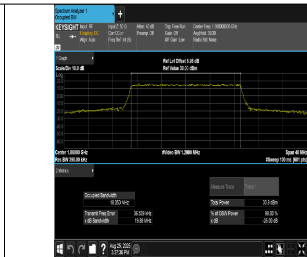
Band2-20MHz-16QAM-18700-100RB#0-PASS
