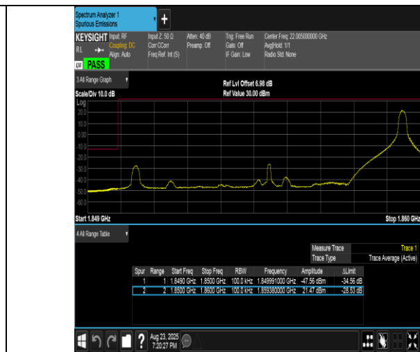
Band2-10MHz-QPSK-18650-1RB#49-PASS
