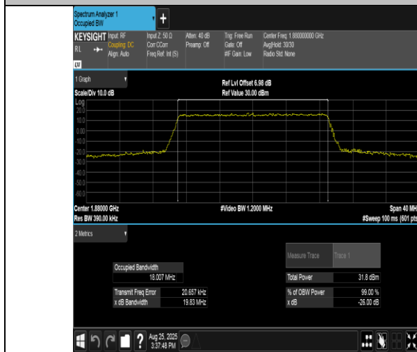
Band2-20MHz-QPSK-18900-100RB#0-PASS
