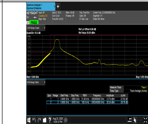
Band2-5MHz-16QAM-18625-1RB#0-PASS
