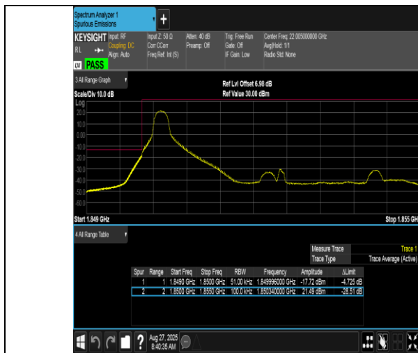
Band2-5MHz-QPSK-18625-1RB#0-PASS
