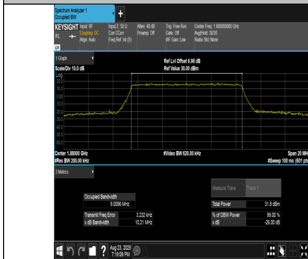
Band2-10MHz-QPSK-18900-50RB#0-PASS
