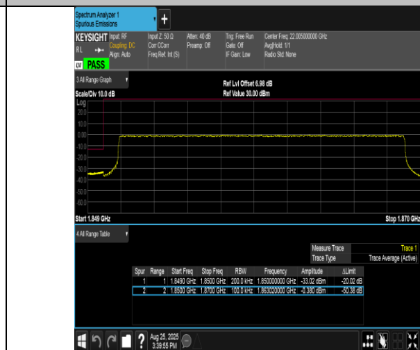
Band2-20MHz-16QAM-18700-100RB#0-PASS
