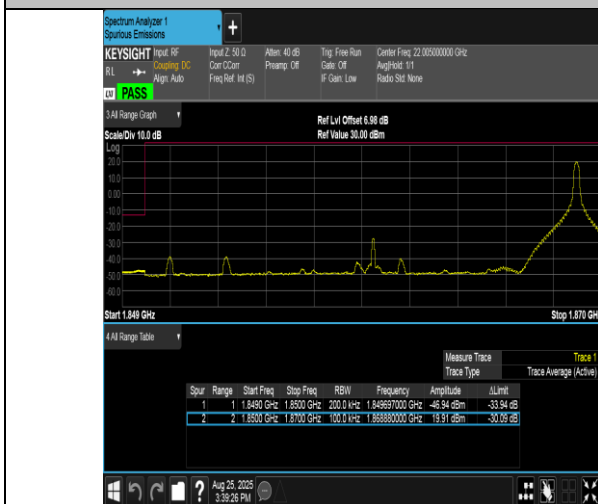
Band2-20MHz-16QAM-18700-1RB#99-PASS
