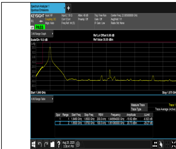
Band2-20MHz-QPSK-18700-1RB#0-PASS
