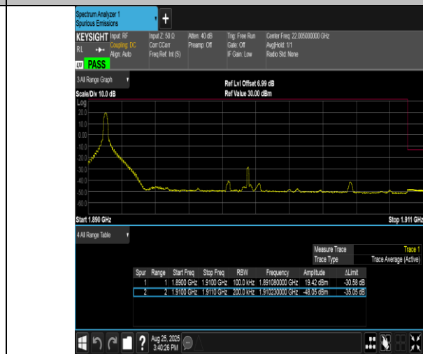
Band2-20MHz-16QAM-19100-1RB#0-PASS
