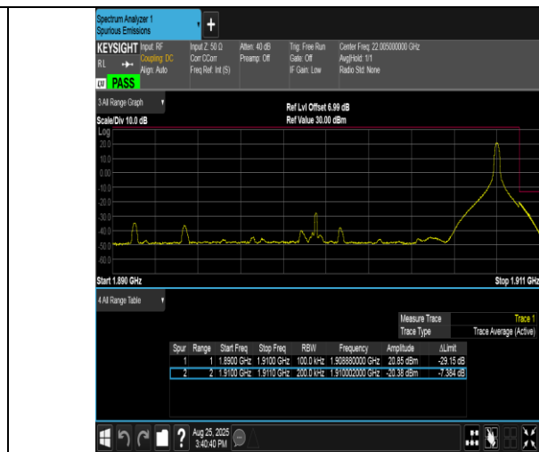
Band2-20MHz-QPSK-19100-1RB#99-PASS
