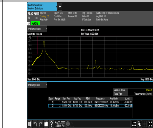
Band2-20MHz-16QAM-18700-1RB#0-PASS
