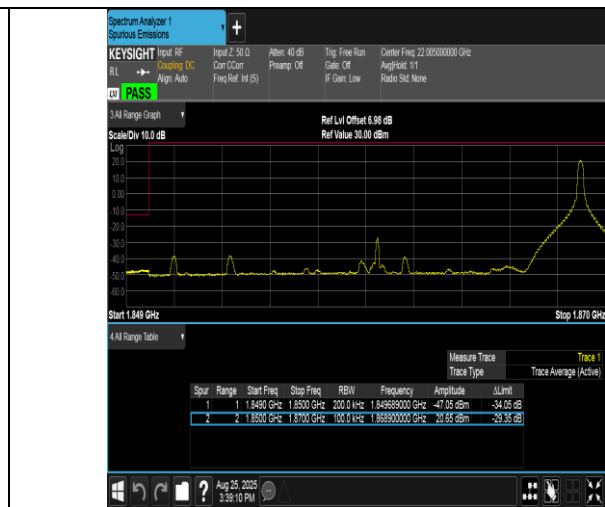
Band2-20MHz-QPSK-18700-1RB#99-PASS
