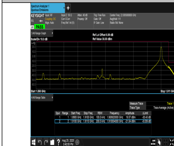
Band2-20MHz-16QAM-19100-1RB#99-PASS
