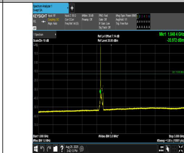
Band2-20MHz-QPSK-18700-1RB#0-1000~3000-PASS
