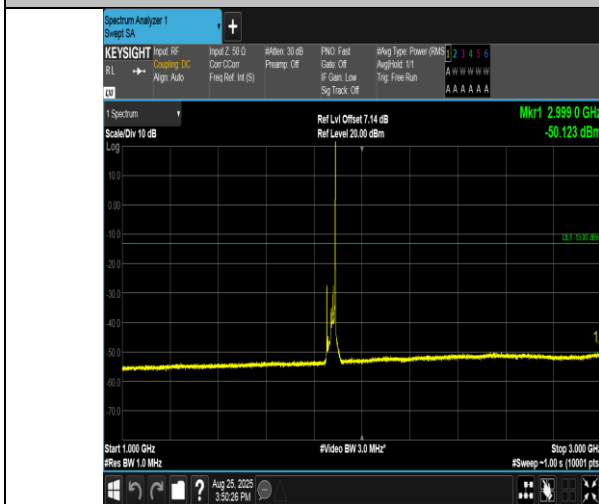
Band2-20MHz-QPSK-18900-1RB#99-1000~3000-PASS
