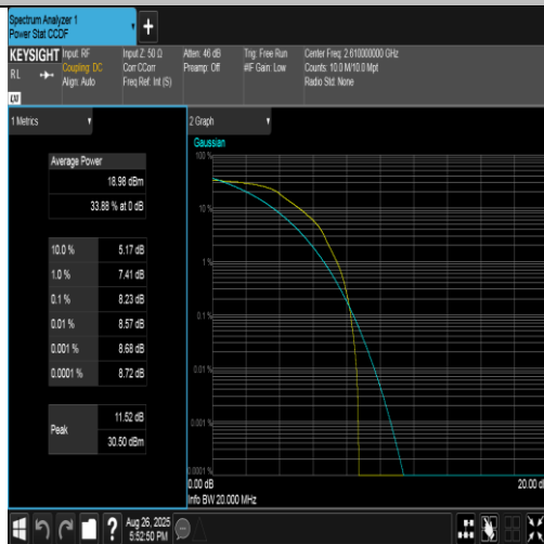
Band38-20MHz-QPSK-38150-1RB#0-PASS
