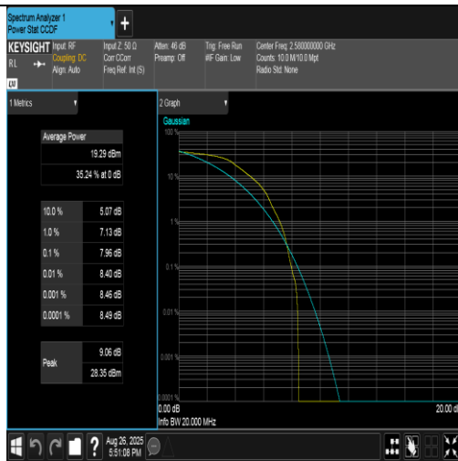
Band38-20MHz-QPSK-37850-1RB#0-PASS
