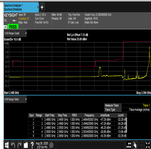
Band38-20MHz-QPSK-37850-1RB#99-PASS
