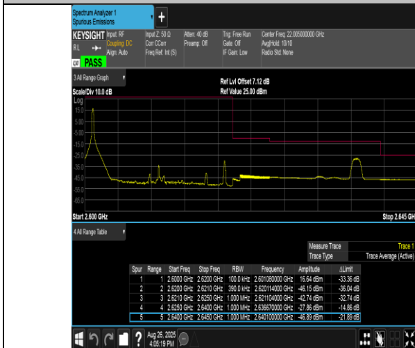
Band38-20MHz-QPSK-38150-1RB#0-PASS
