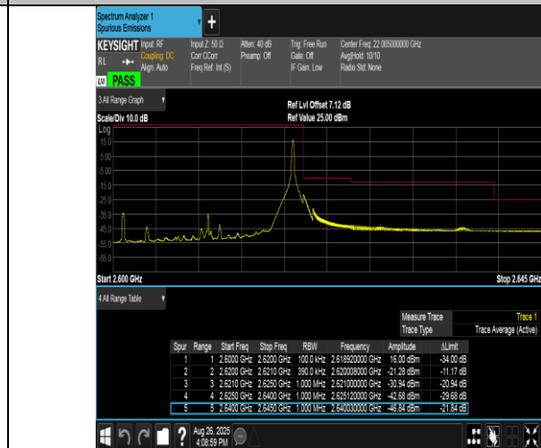
Band38-20MHz-QPSK-38150-1RB#99-PASS
