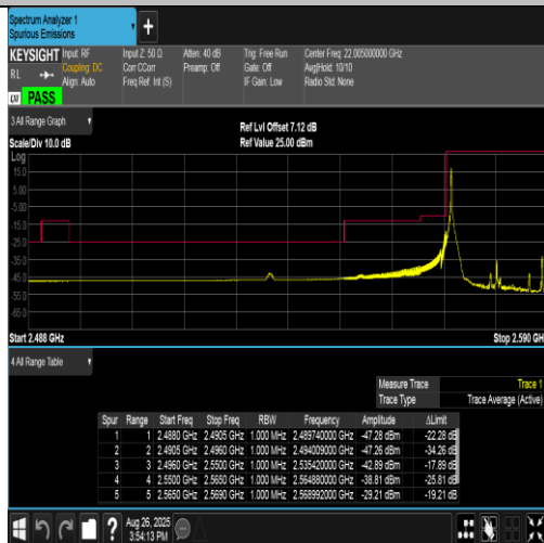
Band38-20MHz-QPSK-37850-1RB#0-PASS
