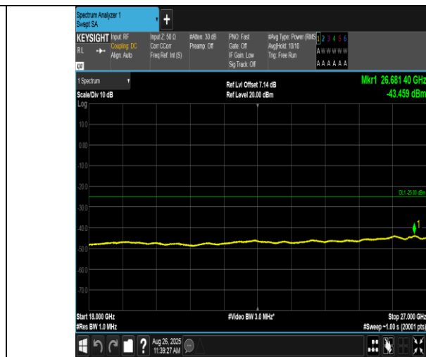
Band38-5MHz-QPSK-38000-25RB#0-18000~27000-PASS
