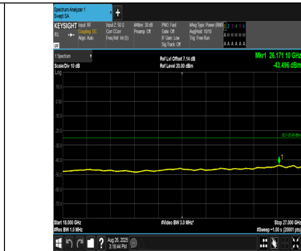
Band38-15MHz-QPSK-38175-1RB#74-18000~27000-PASS
