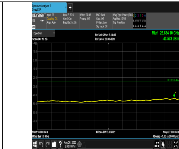
Band38-15MHz-16QAM-38000-1RB#0-18000~27000-PASS
