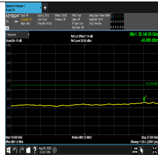
Band38-15MHz-QPSK-38175-1RB#0-18000~27000-PASS
