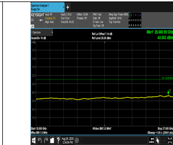
Band38-15MHz-16QAM-37825-1RB#74-18000~27000-PASS
