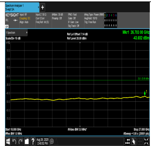
Band38-15MHz-QPSK-38000-1RB#0-18000~27000-PASS
