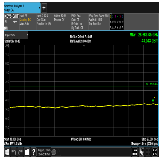
Band38-15MHz-QPSK-38000-1RB#74-18000~27000-PASS
