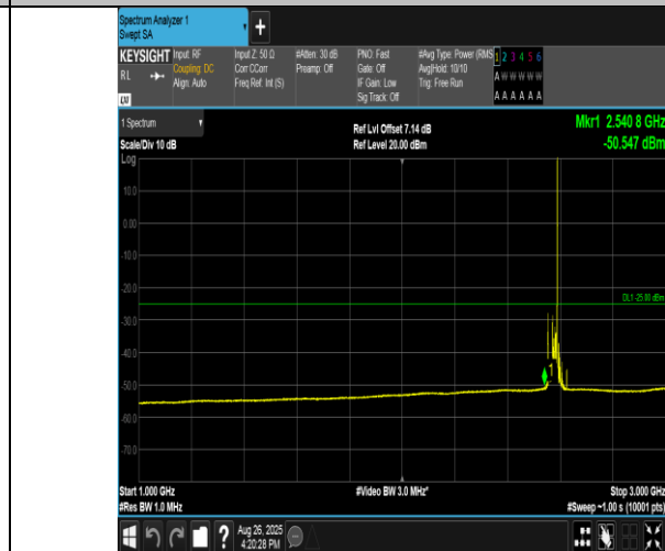
Band38-20MHz-QPSK-37850-1RB#99-1000~3000-PASS
