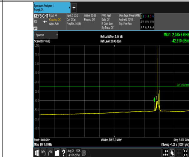
Band38-20MHz-QPSK-37850-1RB#0-1000~3000-PASS
