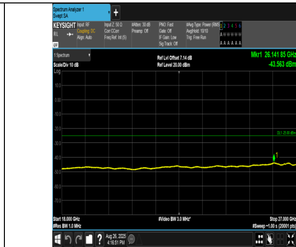
Band38-20MHz-QPSK-37850-1RB#0-18000~27000-PASS
