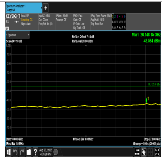
Band38-20MHz-QPSK-38000-1RB#99-18000~27000-PASS
