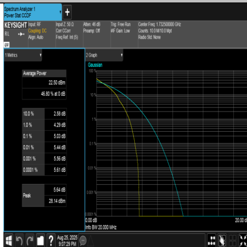
Band4-20MHz-QPSK-20175-1RB#0-PASS
