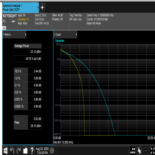
Band4-10MHz-QPSK-20350-1RB#0-PASS
