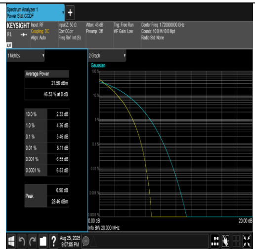
Band4-20MHz-QPSK-20050-100RB#0-PASS
