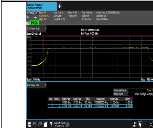
Band4-10MHz-QPSK-20000-50RB#0-PASS
