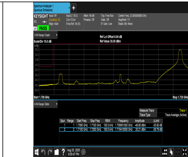
Band4-10MHz-QPSK-20000-1RB#49-PASS
