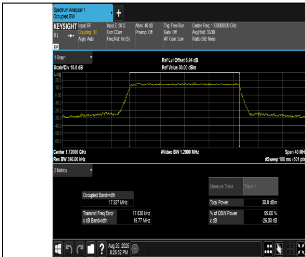
Band4-20MHz-QPSK-20050-100RB#0-PASS
