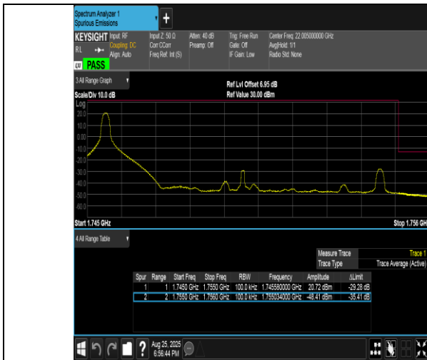
Band4-10MHz-QPSK-20350-1RB#0-PASS
