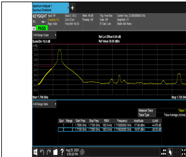
Band4-10MHz-QPSK-20000-1RB#0-PASS
