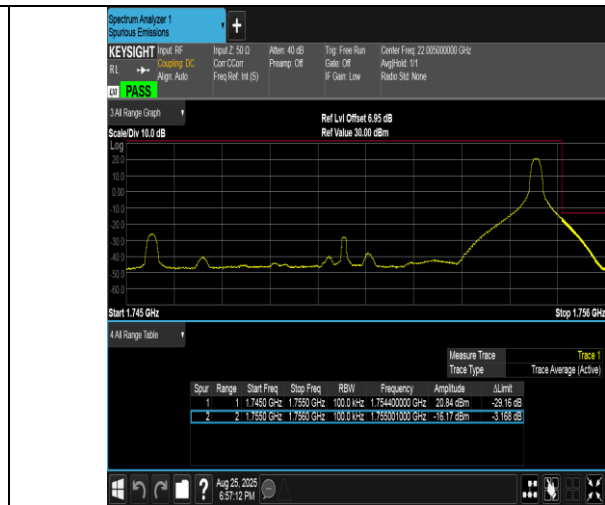
Band4-10MHz-QPSK-20350-1RB#49-PASS
