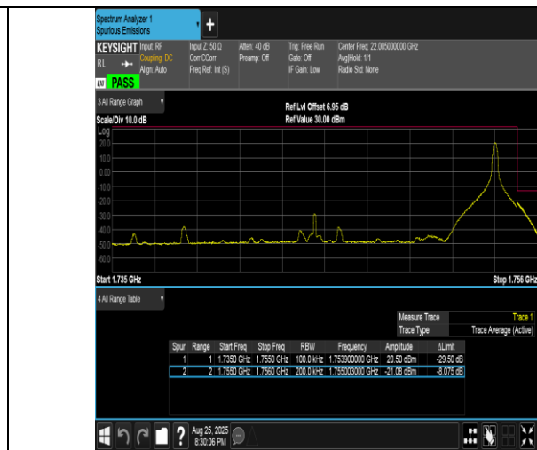
Band4-20MHz-QPSK-20300-1RB#99-PASS
