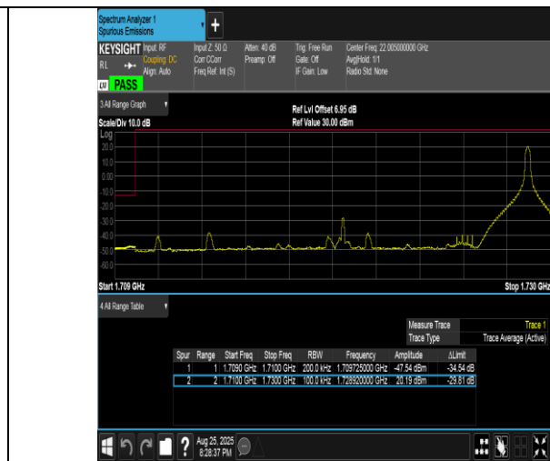
Band4-20MHz-QPSK-20050-1RB#99-PASS
