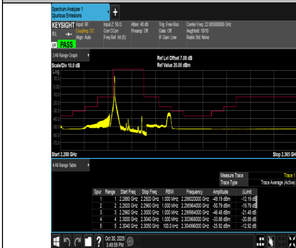
Band40(2305-2315)-10MHz-QPSK-38750-1RB#0-PASS
