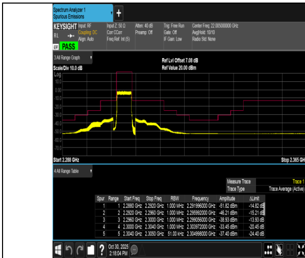
Band40(2305-2315)-5MHz-QPSK-38725-25RB#0-PASS
