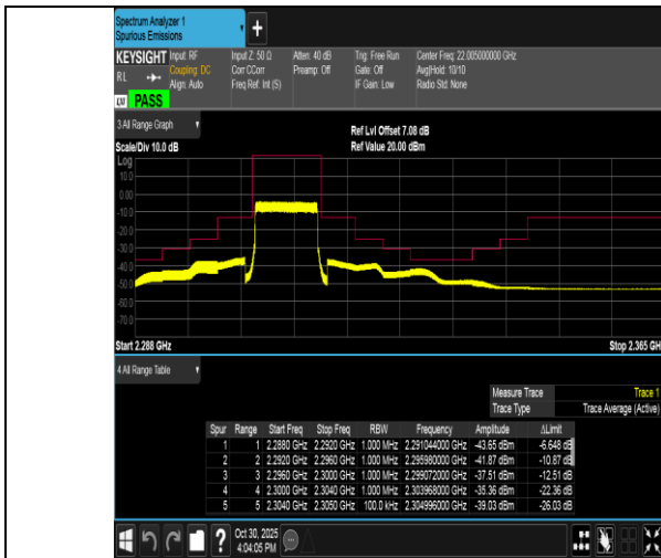
Band40(2305-2315)-10MHz-QPSK-38750-50RB#0-PASS
