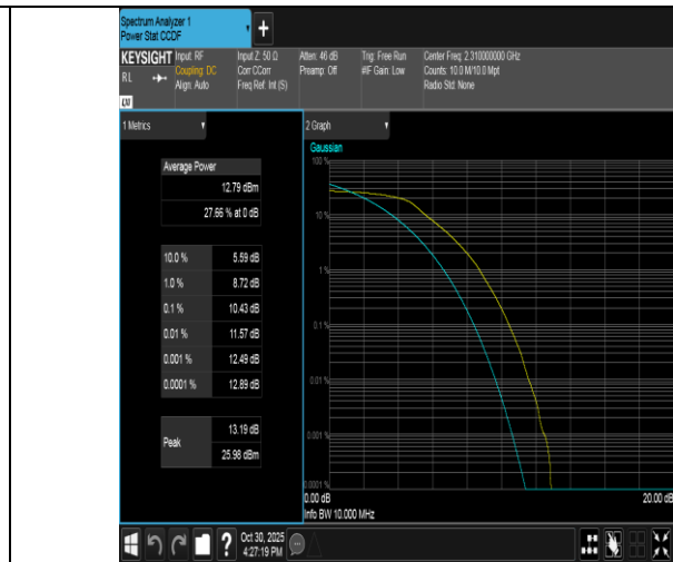
Band40(2305-2315)-10MHz-QPSK-38750-50RB#0-PASS
