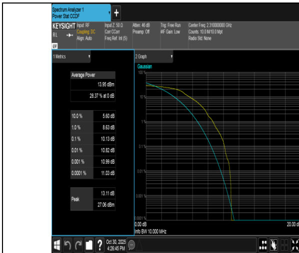
Band40(2305-2315)-10MHz-QPSK-38750-1RB#0-PASS
