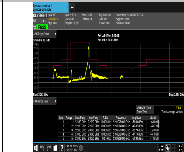
Band40(2305-2315)-10MHz-QPSK-38750-1RB#49-PASS
