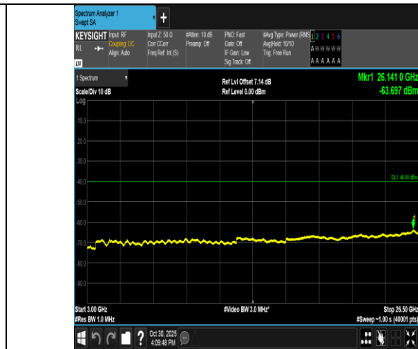
Band40(2305-2315)-10MHz-QPSK-38750-1RB#0-3000~26500-PASS
