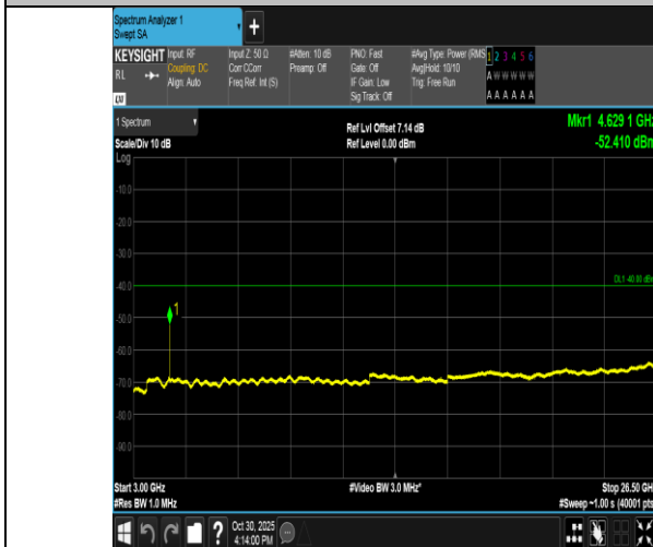
Band40(2305-2315)-10MHz-QPSK-38750-1RB#49-3000~26500-PASS
