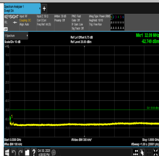
Band40(2305-2315)-10MHz-QPSK-38750-1RB#0-30~1000-PASS
