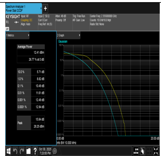
Band40(2350-2360)-10MHz-QPSK-39200-50RB#0-PASS
