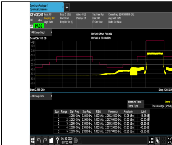
Band40(2350-2360)-10MHz-QPSK-39200-50RB#0-PASS
