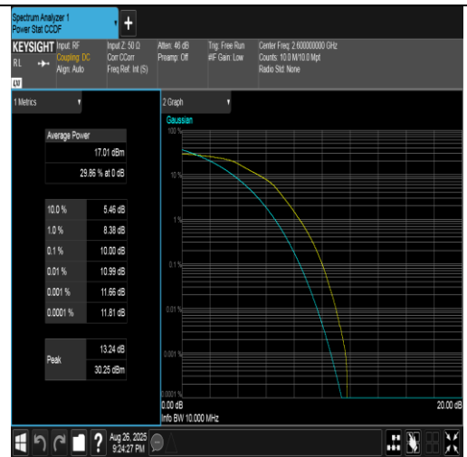
Band41(2555-2655)-10MHz-16QAM-40690-50RB#0-PASS
