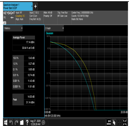
Band41(2555-2655)-20MHz-16QAM-40690-100RB#0-PASS
