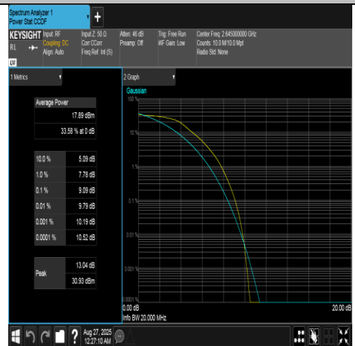
Band41(2555-2655)-20MHz-QPSK-41140-100RB#0-PASS
