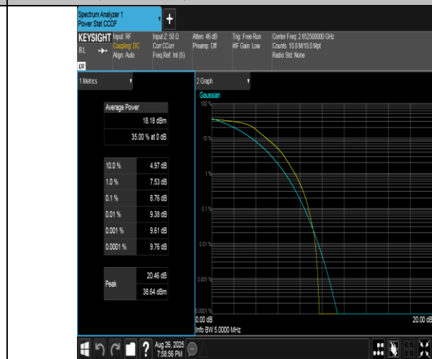
Band41(2555-2655)-5MHz-QPSK-41215-25RB#0-PASS
