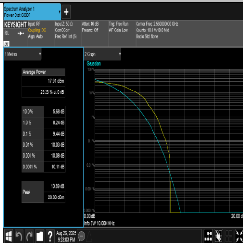
Band41(2555-2655)-10MHz-16QAM-40290-1RB#0-PASS
