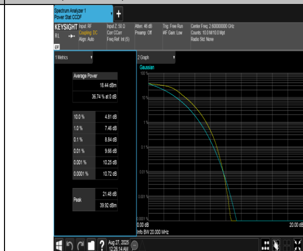
Band41(2555-2655)-20MHz-QPSK-40690-100RB#0-PASS
