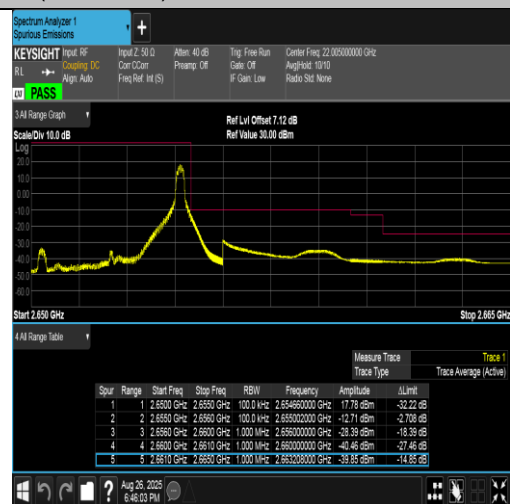
Band41(2555-2655)-5MHz-QPSK-41215-1RB#24-PASS
