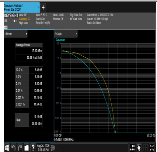
Band41(2555-2655)-10MHz-16QAM-40290-50RB#0-PASS
