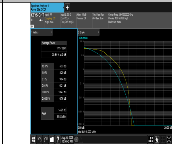
Band41(2555-2655)-15MHz-QPSK-41165-75RB#0-PASS
