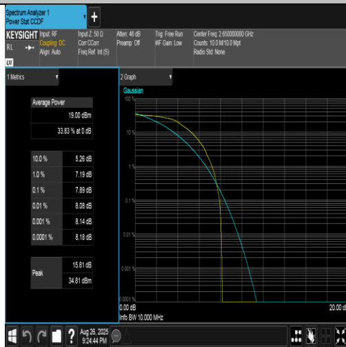
Band41(2555-2655)-10MHz-QPSK-41190-1RB#0-PASS
