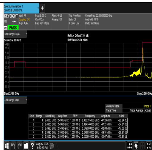
Band41(2555-2655)-5MHz-16QAM-40265-1RB#0-PASS
