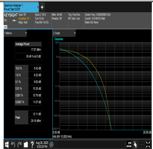
Band41(2555-2655)-10MHz-16QAM-41190-50RB#0-PASS
