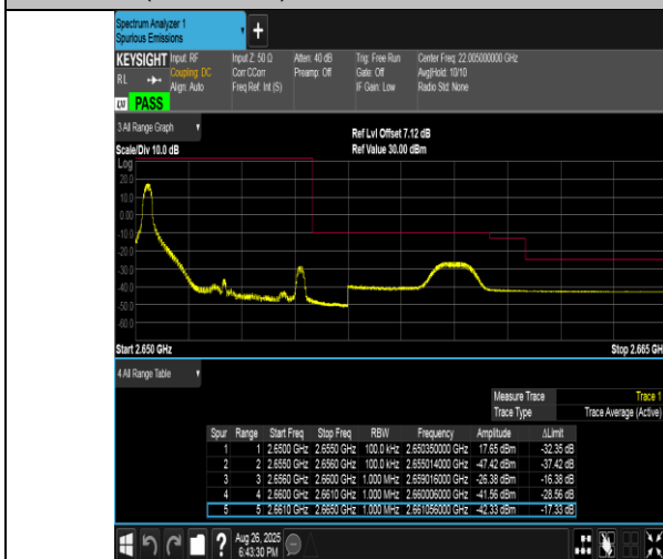
Band41(2555-2655)-5MHz-QPSK-41215-1RB#0-PASS
