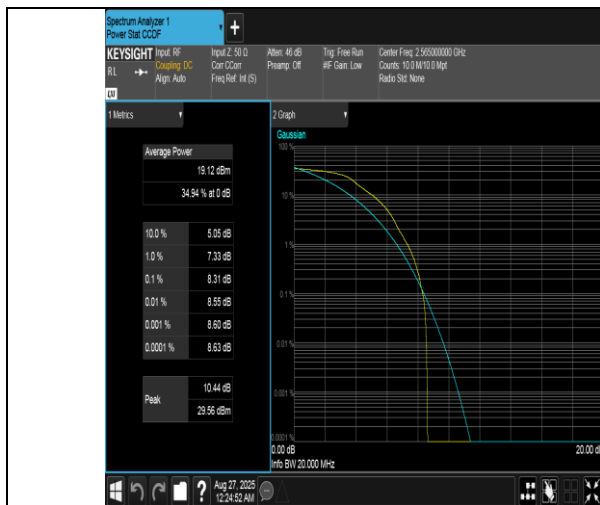
Band41(2555-2655)-20MHz-QPSK-40340-1RB#0-PASS
