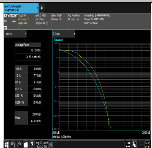
Band41(2555-2655)-10MHz-QPSK-40690-50RB#0-PASS
