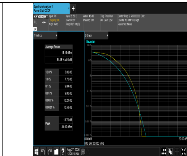
Band41(2555-2655)-20MHz-QPSK-40340-100RB#0-PASS
