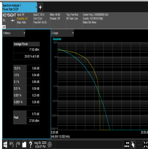
Band41(2555-2655)-10MHz-16QAM-41190-1RB#0-PASS
