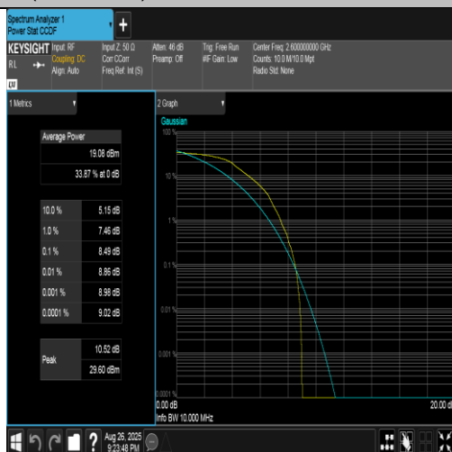
Band41(2555-2655)-10MHz-QPSK-40690-1RB#0-PASS
