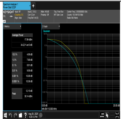
Band41(2555-2655)-10MHz-QPSK-41190-50RB#0-PASS
