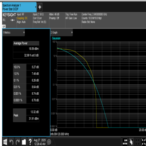
Band41(2555-2655)-20MHz-QPSK-41140-1RB#0-PASS
