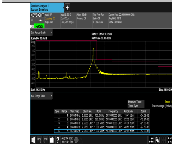
Band41(2555-2655)-20MHz-16QAM-41140-1RB#99-PASS
