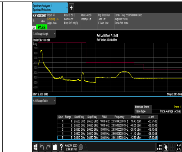
Band41(2555-2655)-5MHz-16QAM-41215-1RB#0-PASS
