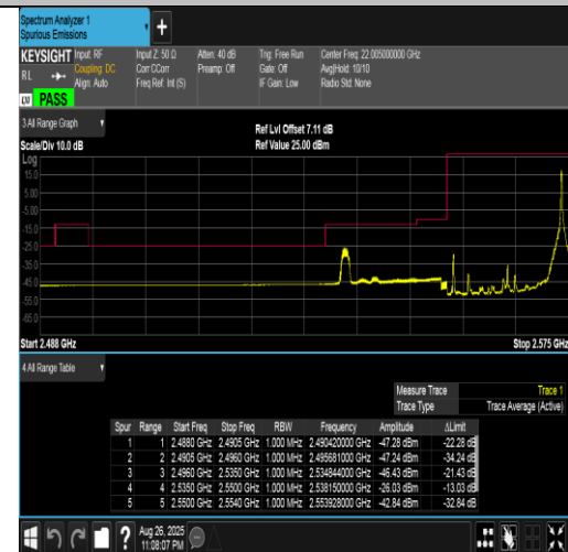
Band41(2555-2655)-20MHz-QPSK-40340-1RB#99-PASS
