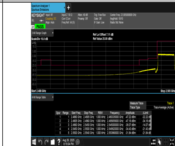
Band41(2555-2655)-10MHz-16QAM-40290-50RB#0-PASS
