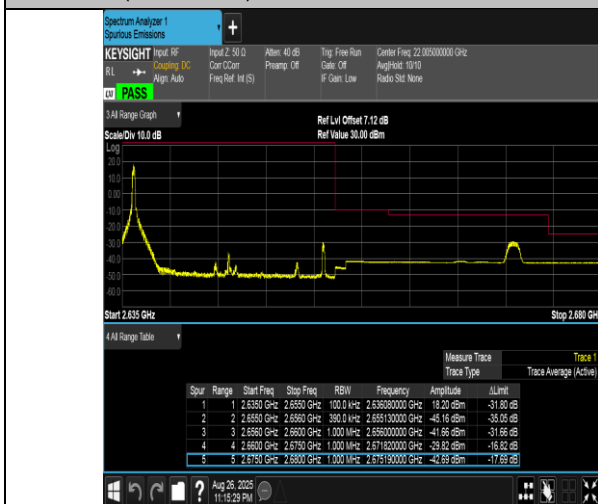
Band41(2555-2655)-20MHz-QPSK-41140-1RB#0-PASS
