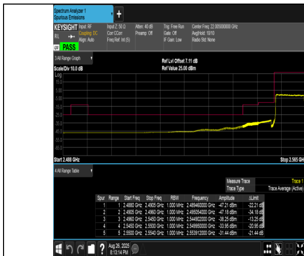
Band41(2555-2655)-10MHz-QPSK-40290-50RB#0-PASS
