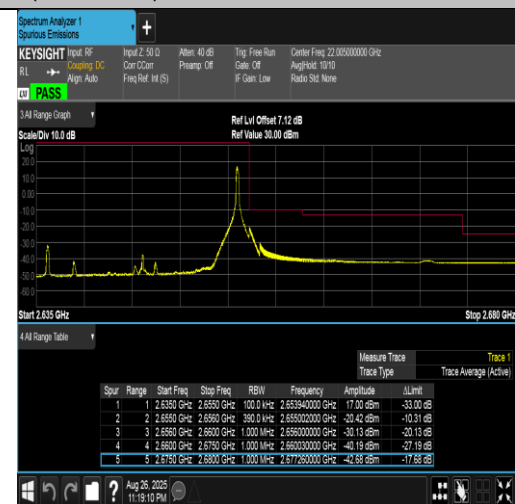
Band41(2555-2655)-20MHz-QPSK-41140-1RB#99-PASS
