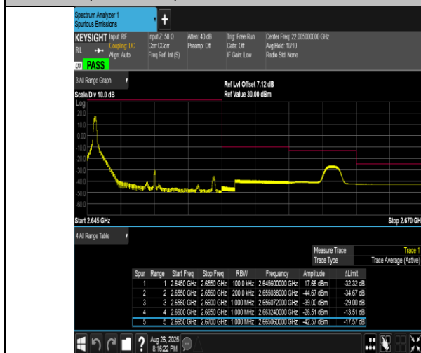
Band41(2555-2655)-10MHz-QPSK-41190-1RB#0-PASS
