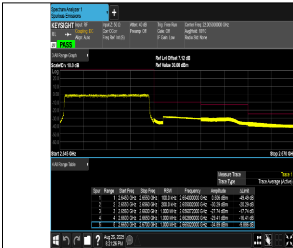
Band41(2555-2655)-10MHz-QPSK-41190-50RB#0-PASS
