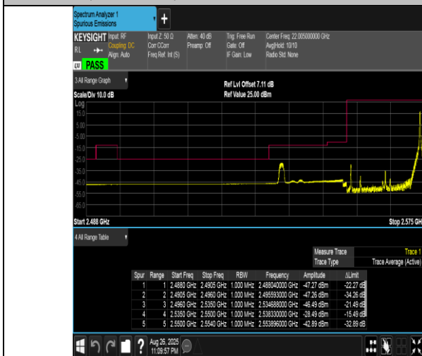
Band41(2555-2655)-20MHz-16QAM-40340-1RB#99-PASS
