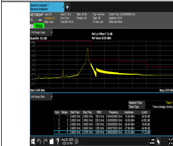
Band41(2555-2655)-10MHz-16QAM-41190-1RB#49-PASS
