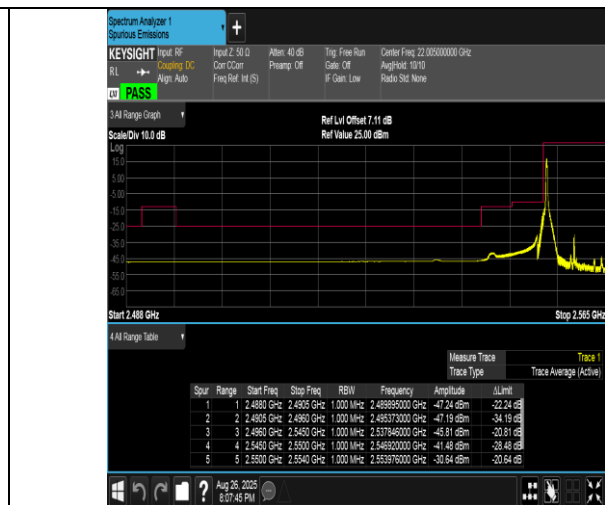
Band41(2555-2655)-10MHz-16QAM-40290-1RB#0-PASS
