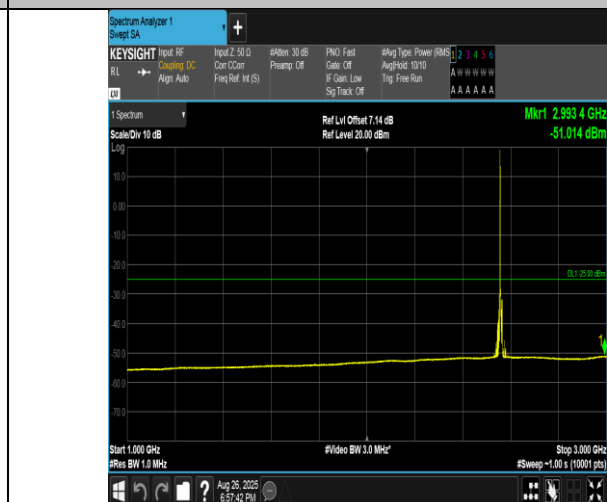
Band41(2555-2655)-5MHz-16QAM-40265-1RB#0-1000~3000-PASS
