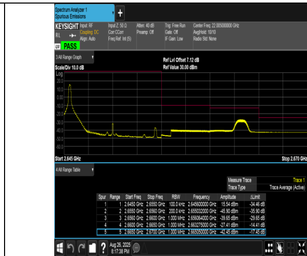
Band41(2555-2655)-10MHz-16QAM-41190-1RB#0-PASS
