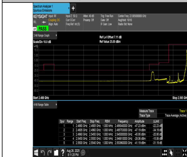
Band41(2555-2655)-10MHz-16QAM-40290-1RB#49-PASS
