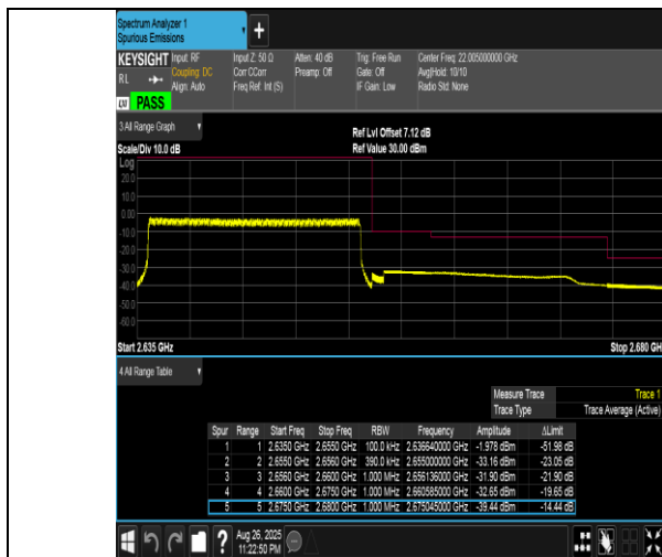
Band41(2555-2655)-20MHz-QPSK-41140-100RB#0-PASS
