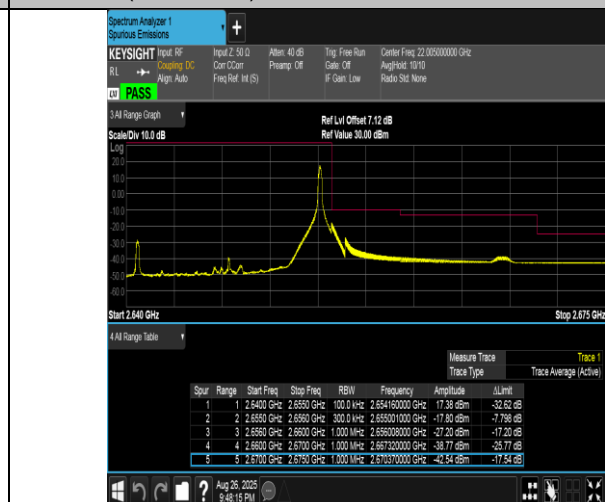
Band41(2555-2655)-15MHz-QPSK-41165-1RB#74-PASS
