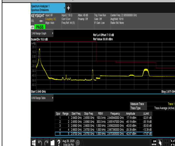
Band41(2555-2655)-15MHz-QPSK-41165-1RB#0-PASS
