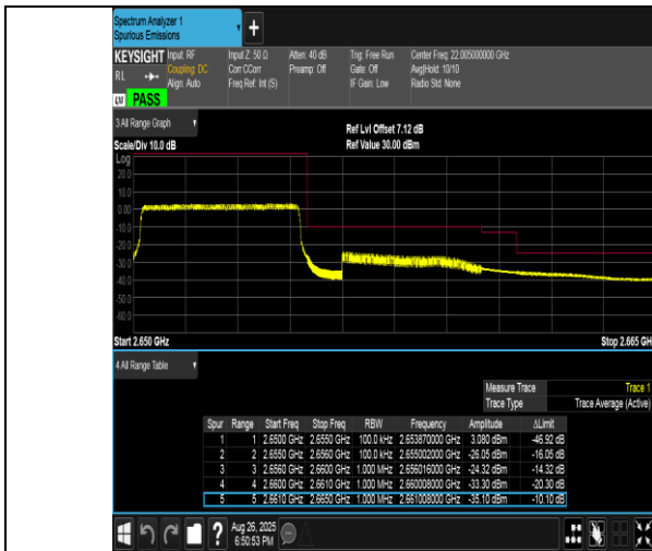
Band41(2555-2655)-5MHz-QPSK-41215-25RB#0-PASS
