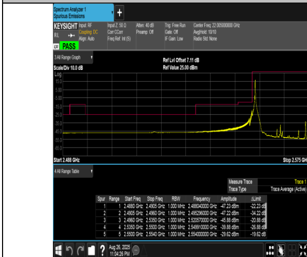
Band41(2555-2655)-20MHz-QPSK-40340-1RB#0-PASS
