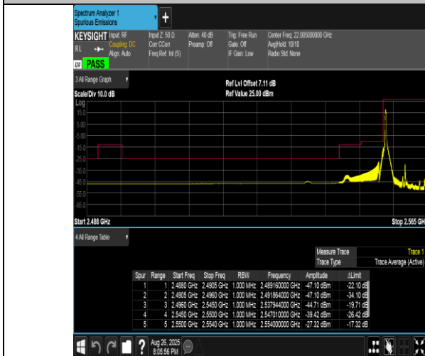
Band41(2555-2655)-10MHz-QPSK-40290-1RB#0-PASS
