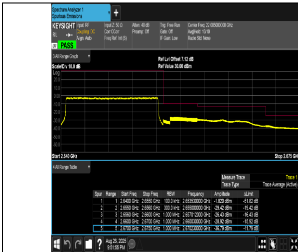
Band41(2555-2655)-15MHz-QPSK-41165-75RB#0-PASS
