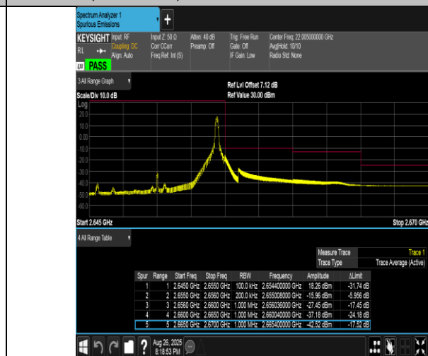
Band41(2555-2655)-10MHz-QPSK-41190-1RB#49-PASS
