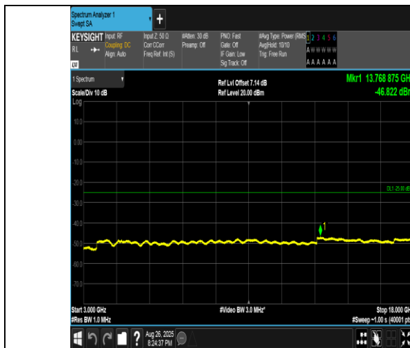
Band41(2555-2655)-10MHz-QPSK-40290-1RB#0-3000~18000-PASS
