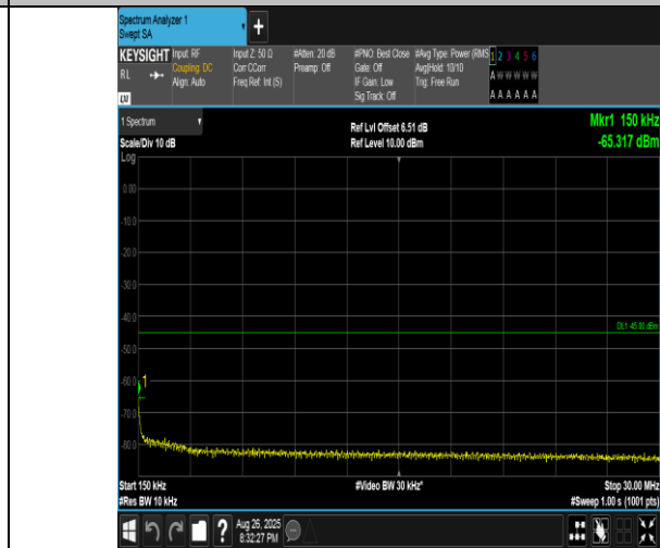
Band41(2555-2655)-10MHz-QPSK-40290-50RB#0-0.15~30-PASS
