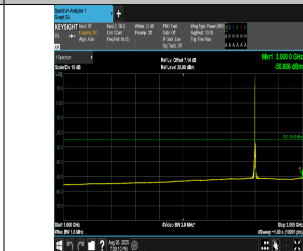
Band41(2555-2655)-5MHz-QPSK-40690-1RB#0-1000~3000-PASS
