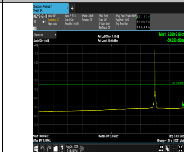
Band41(2555-2655)-5MHz-QPSK-40690-25RB#0-1000~3000-PASS
