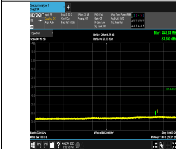
Band41(2555-2655)-10MHz-QPSK-40290-50RB#0-30~1000-PASS
