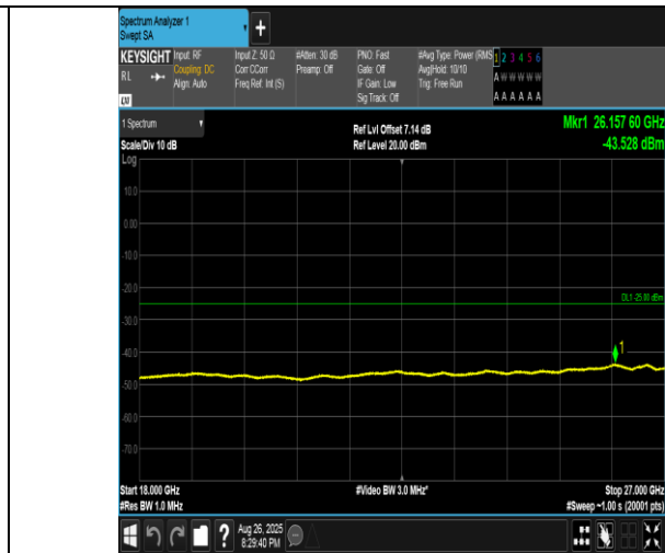
Band41(2555-2655)-10MHz-QPSK-40290-1RB#49-18000~27000-PASS
