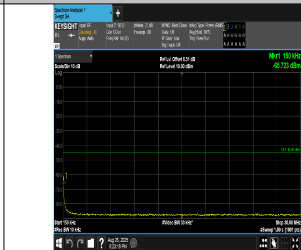
Band41(2555-2655)-10MHz-QPSK-40290-1RB#0-0.15~30-PASS
