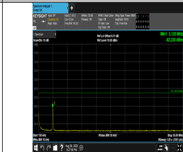
Band41(2555-2655)-10MHz-QPSK-40290-1RB#49-0.15~30-PASS
