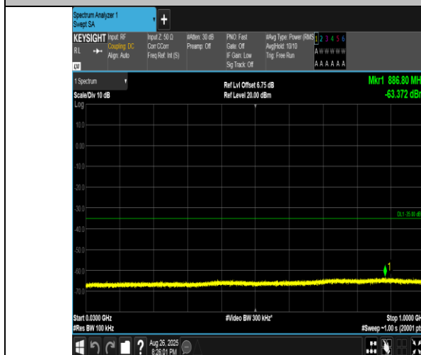
Band41(2555-2655)-10MHz-16QAM-40290-1RB#0-30~1000-PASS
