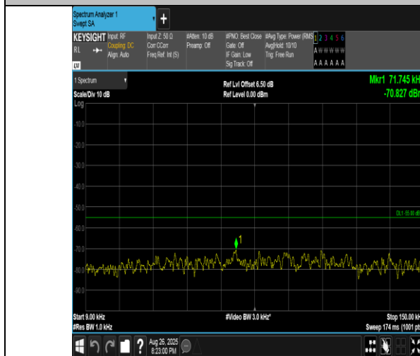
Band41(2555-2655)-10MHz-QPSK-40290-1RB#0-0.009~0.15-PASS
