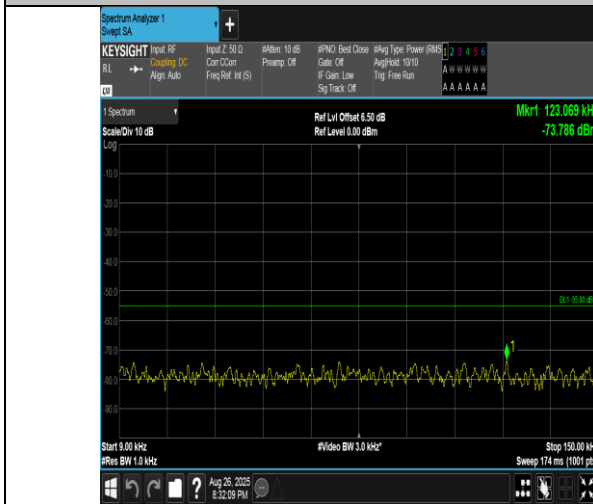
Band41(2555-2655)-10MHz-QPSK-40290-50RB#0-0.009~0.15-PASS
