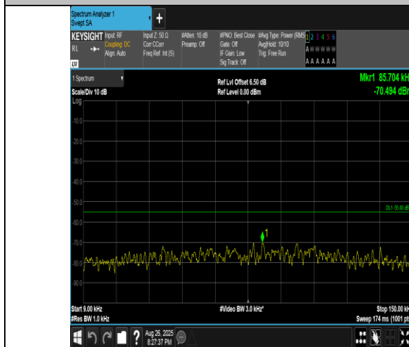
Band41(2555-2655)-10MHz-QPSK-40290-1RB#49-0.009~0.15-PASS
