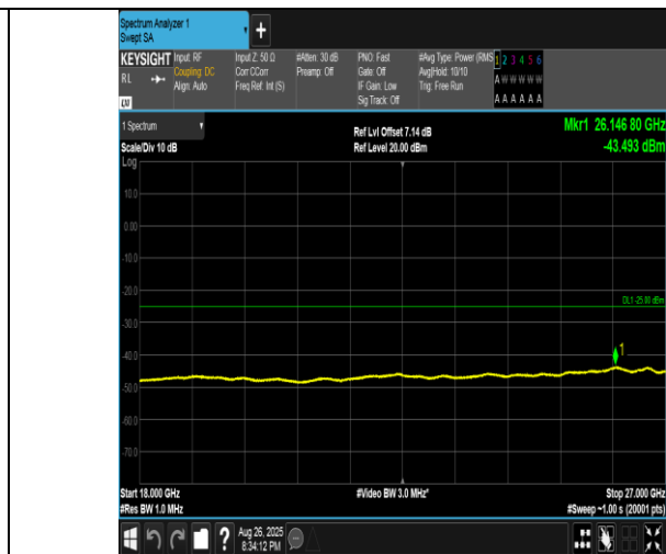
Band41(2555-2655)-10MHz-QPSK-40290-50RB#0-18000~27000-PASS
