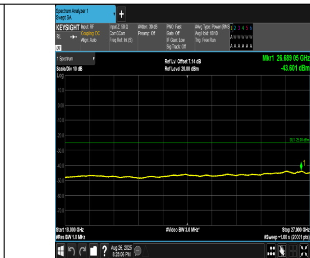
Band41(2555-2655)-10MHz-QPSK-40290-1RB#0-18000~27000-PASS
