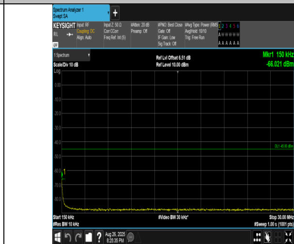
Band41(2555-2655)-10MHz-16QAM-40290-1RB#0-0.15~30-PASS
