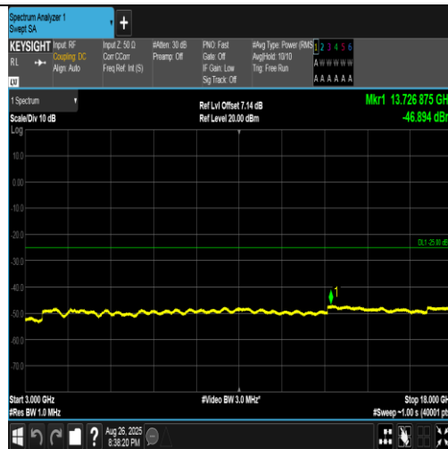
Band41(2555-2655)-10MHz-QPSK-40690-1RB#0-3000~18000-PASS
