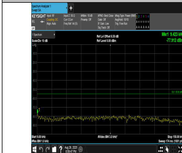
Band41(2555-2655)-10MHz-QPSK-41190-50RB#0-0.009~0.15-PASS
