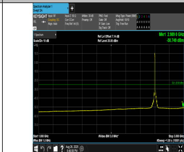
Band41(2555-2655)-10MHz-QPSK-40690-50RB#0-1000~3000-PASS
