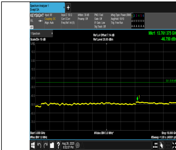
Band41(2555-2655)-10MHz-QPSK-41190-1RB#0-3000~18000-PASS
