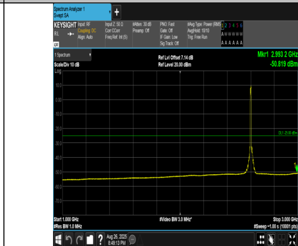
Band41(2555-2655)-10MHz-16QAM-40690-50RB#0-1000~3000-PASS
