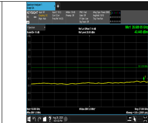
Band41(2555-2655)-10MHz-QPSK-41190-50RB#0-18000~27000-PASS
