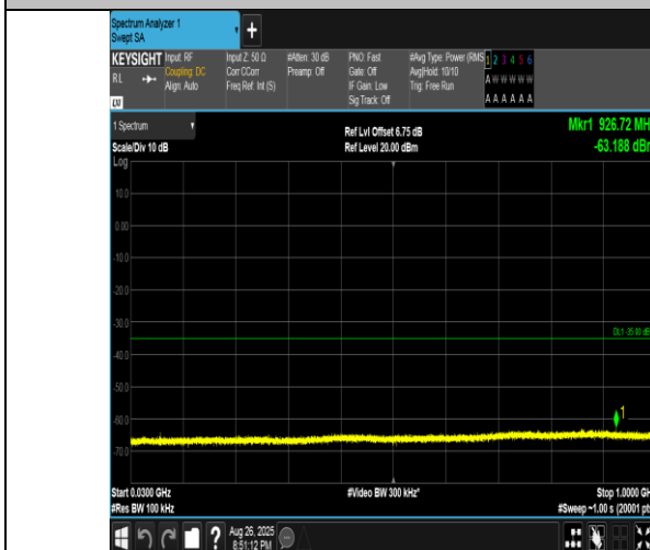
Band41(2555-2655)-10MHz-QPSK-41190-1RB#0-30~1000-PASS
