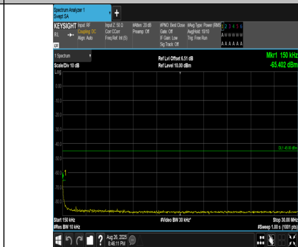
Band41(2555-2655)-10MHz-QPSK-40690-50RB#0-0.15~30-PASS
