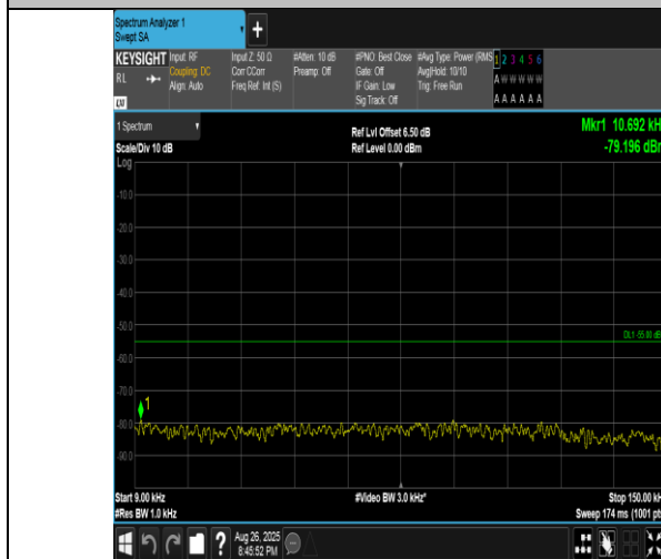
Band41(2555-2655)-10MHz-QPSK-40690-50RB#0-0.009~0.15-PASS
