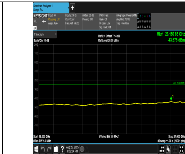
Band41(2555-2655)-10MHz-QPSK-41190-1RB#0-18000~27000-PASS
