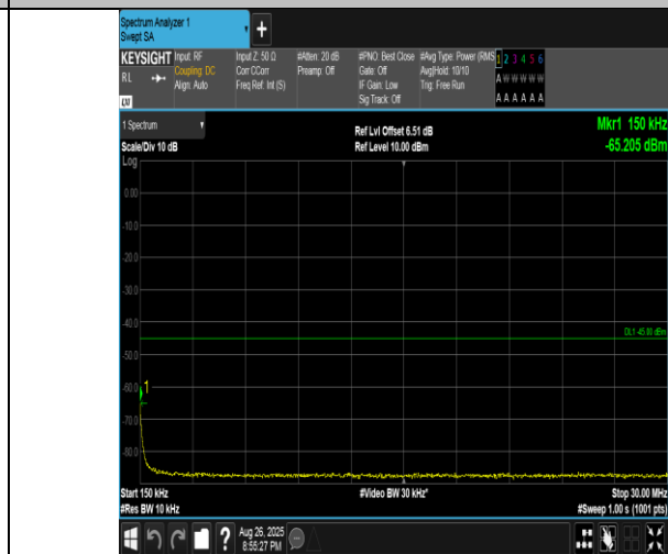
Band41(2555-2655)-10MHz-QPSK-41190-1RB#49-0.15~30-PASS
