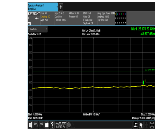
Band41(2555-2655)-10MHz-QPSK-40690-50RB#0-18000~27000-PASS
