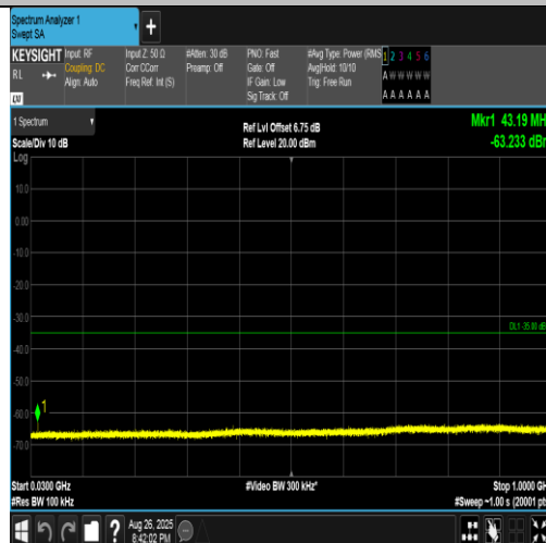
Band41(2555-2655)-10MHz-QPSK-40690-1RB#49-30~1000-PASS
