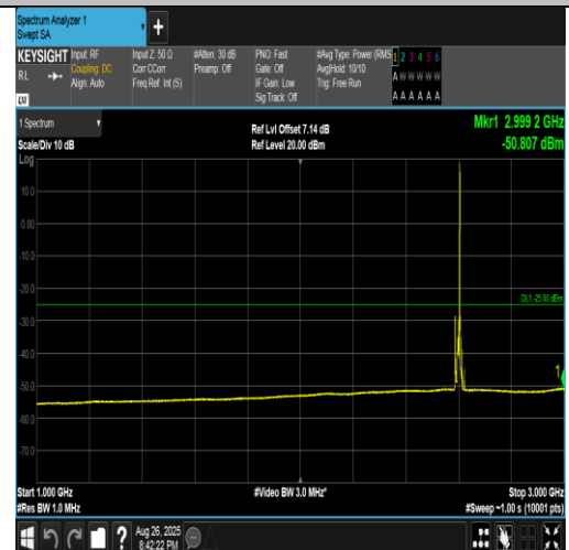
Band41(2555-2655)-10MHz-QPSK-40690-1RB#49-1000~3000-PASS
