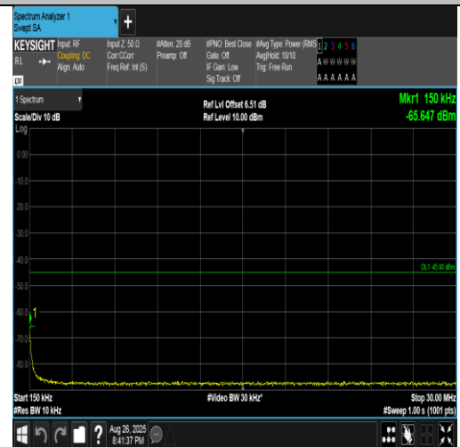
Band41(2555-2655)-10MHz-QPSK-40690-1RB#49-0.15~30-PASS
