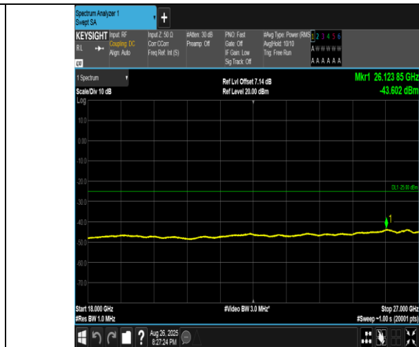
Band41(2555-2655)-10MHz-16QAM-40290-1RB#0-18000~27000-PASS
