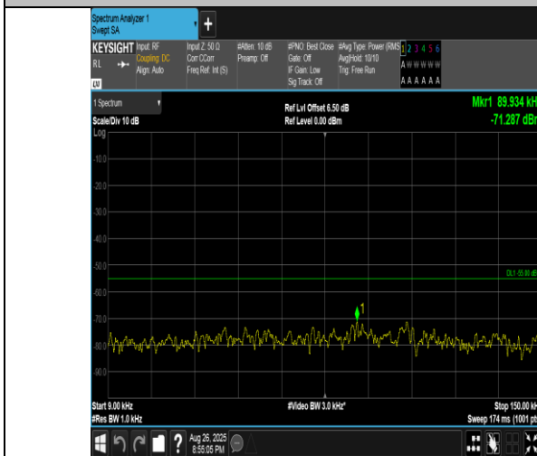
Band41(2555-2655)-10MHz-QPSK-41190-1RB#49-0.009~0.15-PASS
