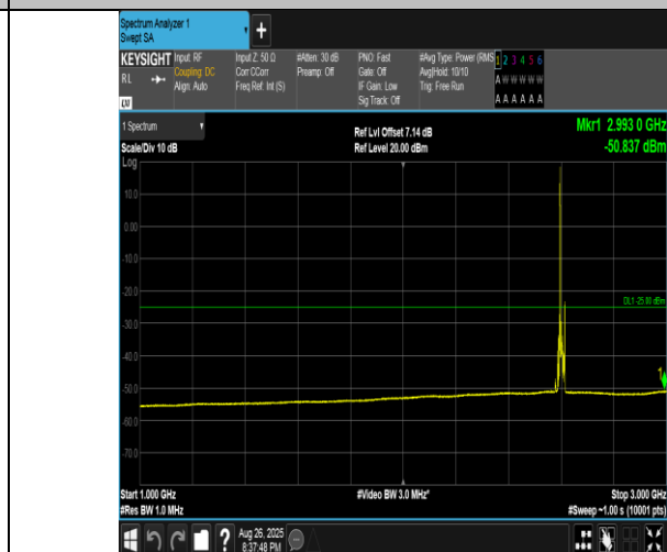
Band41(2555-2655)-10MHz-QPSK-40690-1RB#0-1000~3000-PASS
