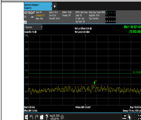
Band41(2555-2655)-10MHz-QPSK-41190-1RB#0-0.009~0.15-PASS
