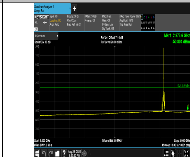
Band41(2555-2655)-10MHz-16QAM-41190-1RB#0-1000~3000-PASS
