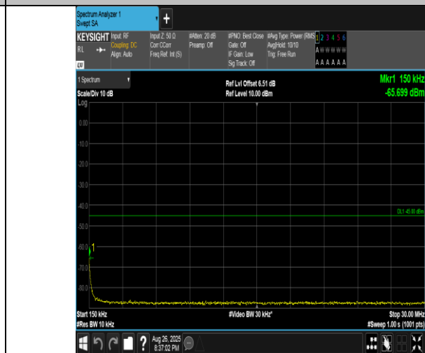
Band41(2555-2655)-10MHz-QPSK-40690-1RB#0-0.15~30-PASS
