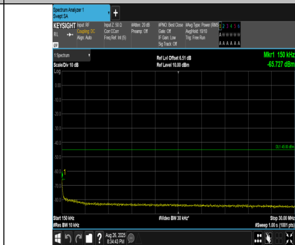
Band41(2555-2655)-10MHz-16QAM-40290-50RB#0-0.15~30-PASS
