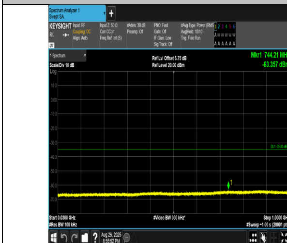
Band41(2555-2655)-10MHz-QPSK-41190-1RB#49-30~1000-PASS
