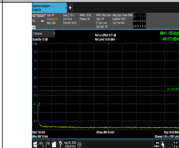
Band41(2555-2655)-10MHz-QPSK-41190-50RB#0-0.15~30-PASS
