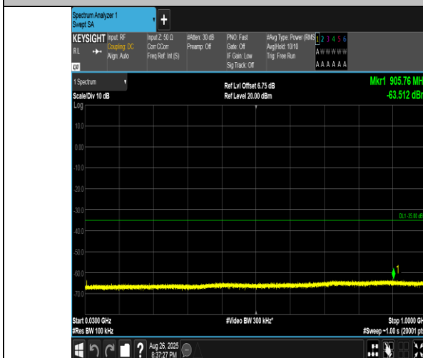
Band41(2555-2655)-10MHz-QPSK-40690-1RB#0-30~1000-PASS
