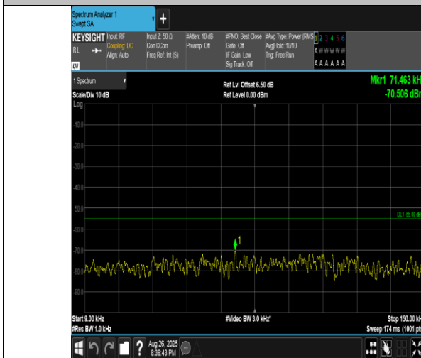
Band41(2555-2655)-10MHz-QPSK-40690-1RB#0-0.009~0.15-PASS
