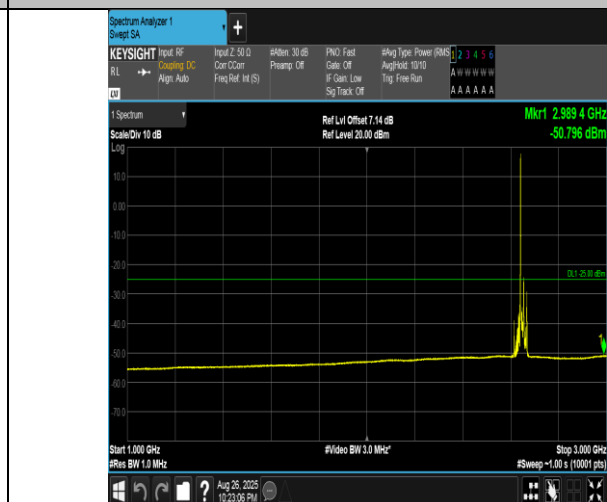
Band41(2555-2655)-15MHz-QPSK-41165-1RB#0-1000~3000-PASS
