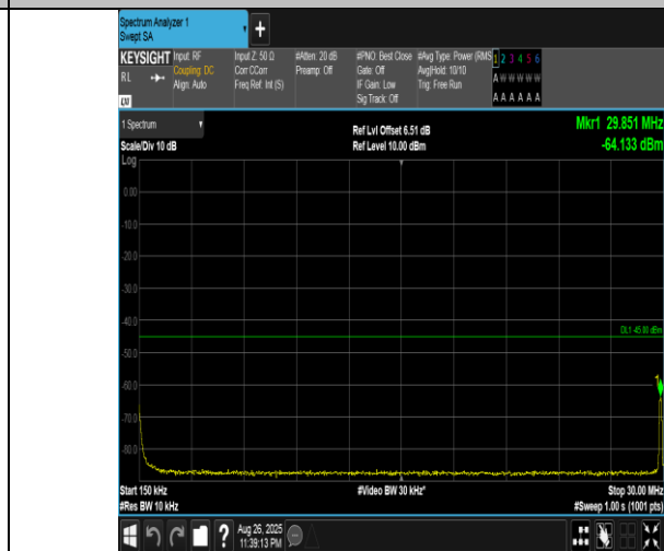
Band41(2555-2655)-20MHz-QPSK-40690-1RB#0-0.15~30-PASS
