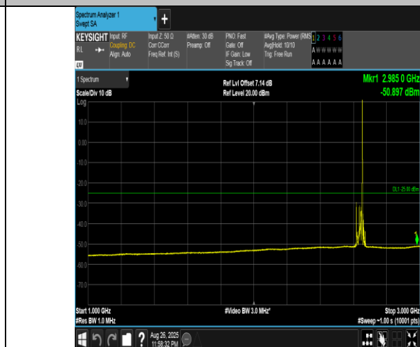
Band41(2555-2655)-20MHz-QPSK-41140-1RB#99-1000~3000-PASS
