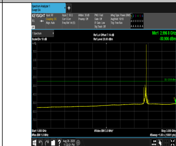
Band41(2555-2655)-20MHz-16QAM-40340-1RB#99-1000~3000-PASS
