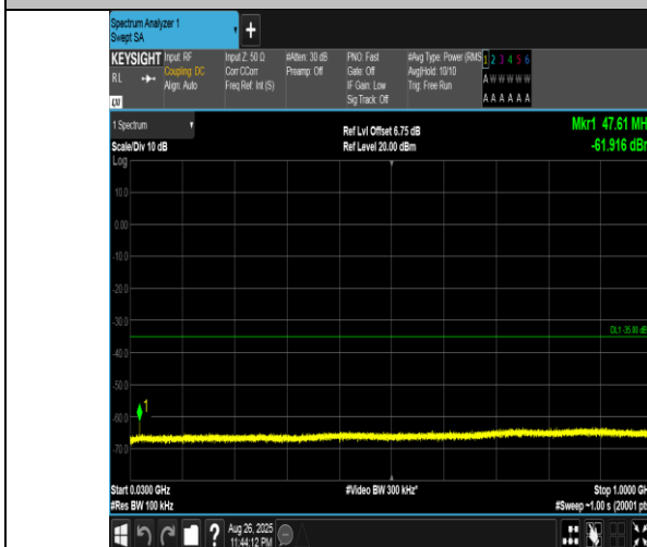
Band41(2555-2655)-20MHz-QPSK-40690-1RB#99-30~1000-PASS
