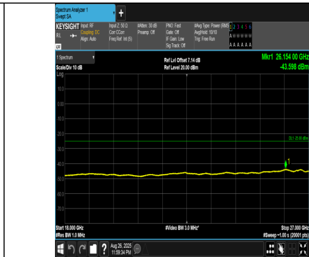
Band41(2555-2655)-20MHz-QPSK-41140-1RB#99-18000~27000-PASS
