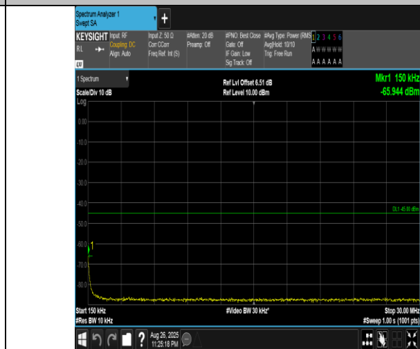
Band41(2555-2655)-20MHz-QPSK-40340-1RB#0-0.15~30-PASS
