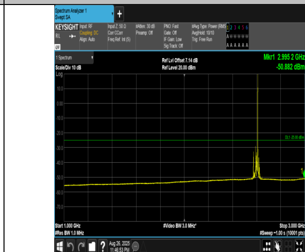
Band41(2555-2655)-20MHz-16QAM-40690-1RB#99-1000~3000-PASS
