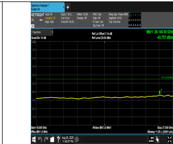
Band41(2555-2655)-20MHz-QPSK-40690-1RB#0-18000~27000-PASS
