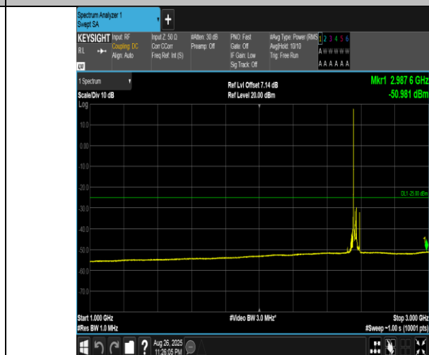
Band41(2555-2655)-20MHz-QPSK-40340-1RB#0-1000~3000-PASS
