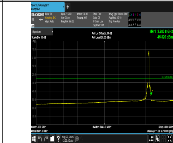
Band41(2555-2655)-20MHz-QPSK-41140-100RB#0-1000~3000-PASS
