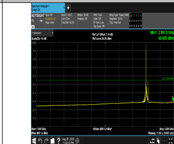
Band41(2555-2655)-20MHz-16QAM-40690-1RB#0-1000~3000-PASS
