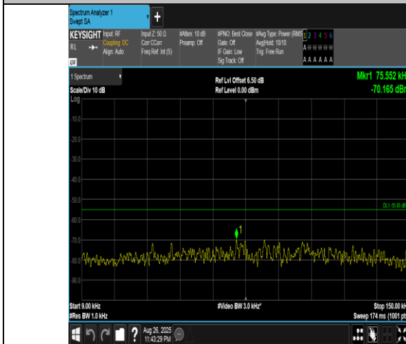
Band41(2555-2655)-20MHz-QPSK-40690-1RB#99-0.009~0.15-PASS
