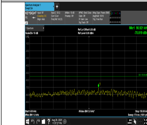
Band41(2555-2655)-20MHz-QPSK-41140-1RB#99-0.009~0.15-PASS
