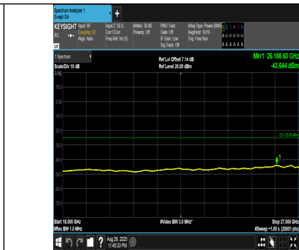
Band41(2555-2655)-20MHz-QPSK-40690-1RB#99-18000~27000-PASS
