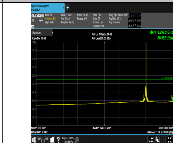
Band41(2555-2655)-20MHz-QPSK-40690-1RB#99-1000~3000-PASS
