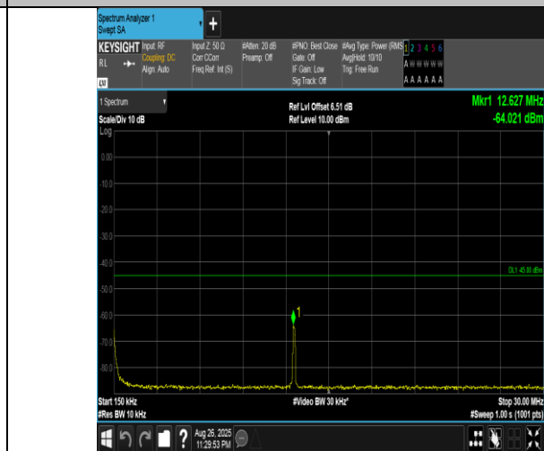
Band41(2555-2655)-20MHz-QPSK-40340-1RB#99-0.15~30-PASS
