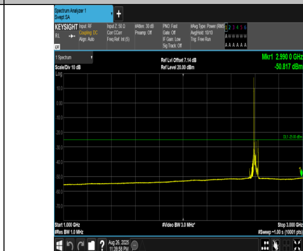
Band41(2555-2655)-20MHz-QPSK-40690-1RB#0-1000~3000-PASS
