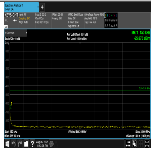
Band41(2555-2655)-20MHz-QPSK-41140-1RB#0-0.15~30-PASS
