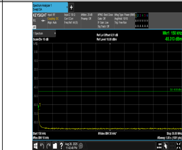
Band41(2555-2655)-20MHz-QPSK-40690-1RB#99-0.15~30-PASS
