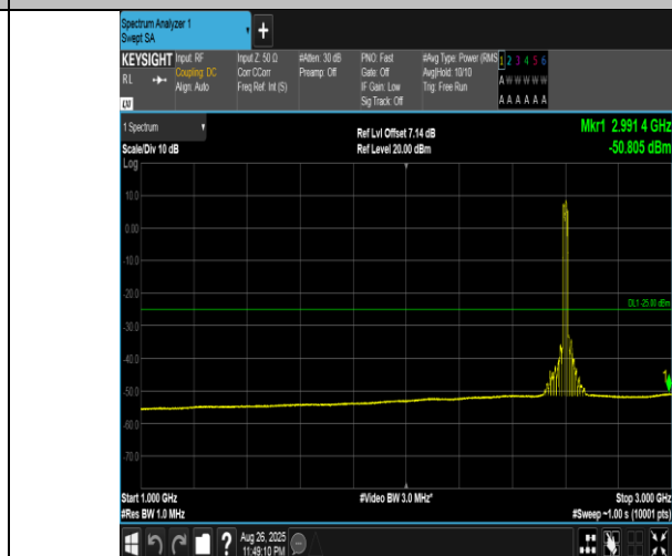
Band41(2555-2655)-20MHz-QPSK-40690-100RB#0-1000~3000-PASS
