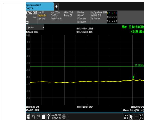
Band41(2555-2655)-20MHz-QPSK-40340-1RB#99-18000~27000-PASS
