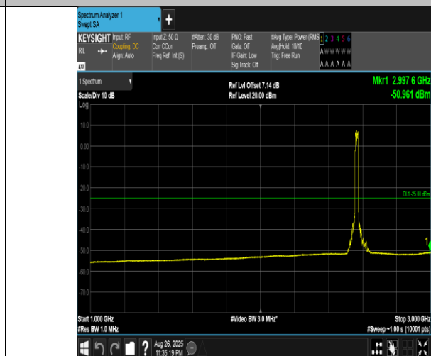
Band41(2555-2655)-20MHz-QPSK-40340-100RB#0-1000~3000-PASS
