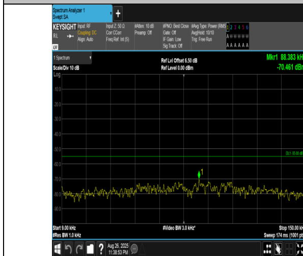
Band41(2555-2655)-20MHz-QPSK-40690-1RB#0-0.009~0.15-PASS
