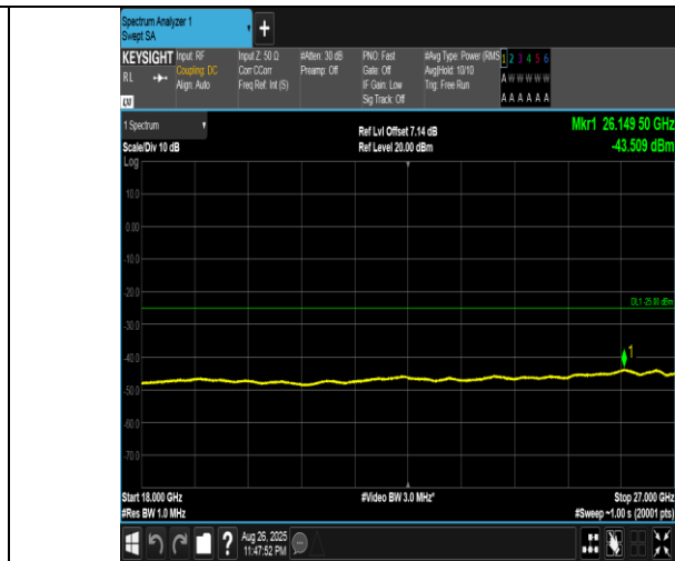
Band41(2555-2655)-20MHz-16QAM-40690-1RB#99-18000~27000-PASS
