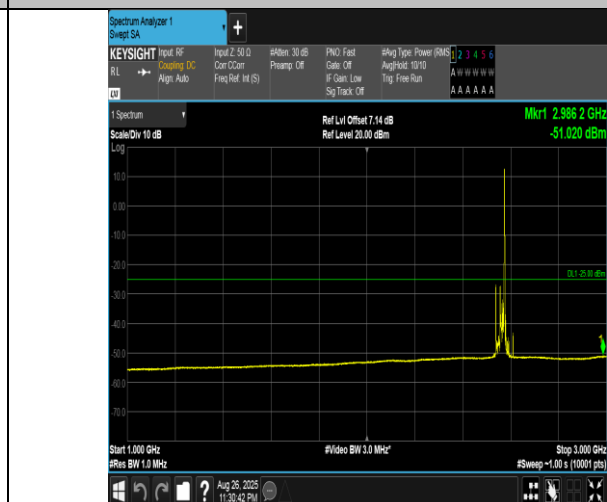
Band41(2555-2655)-20MHz-QPSK-40340-1RB#99-1000~3000-PASS
