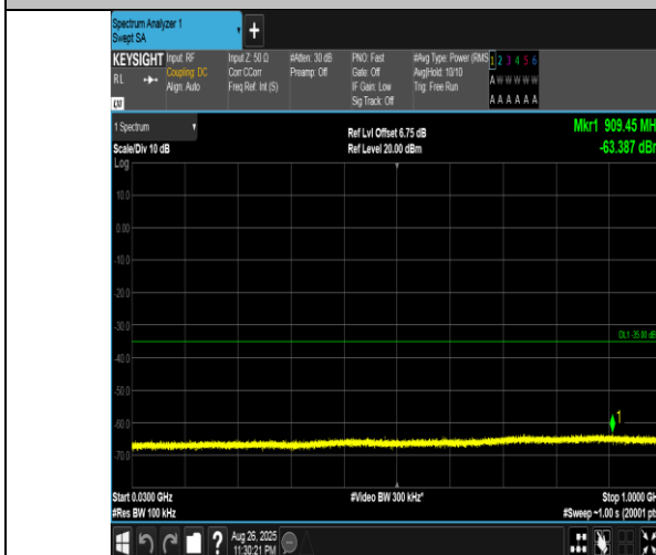
Band41(2555-2655)-20MHz-QPSK-40340-1RB#99-30~1000-PASS
