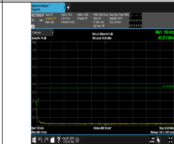
Band41(2555-2655)-20MHz-QPSK-41140-1RB#99-0.15~30-PASS
