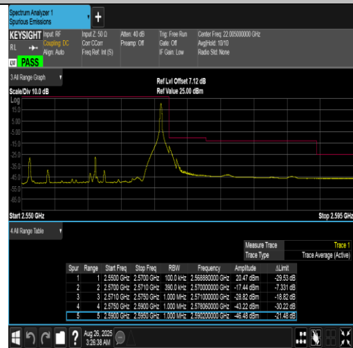
Band7-20MHz-QPSK-21350-1RB#99-PASS
