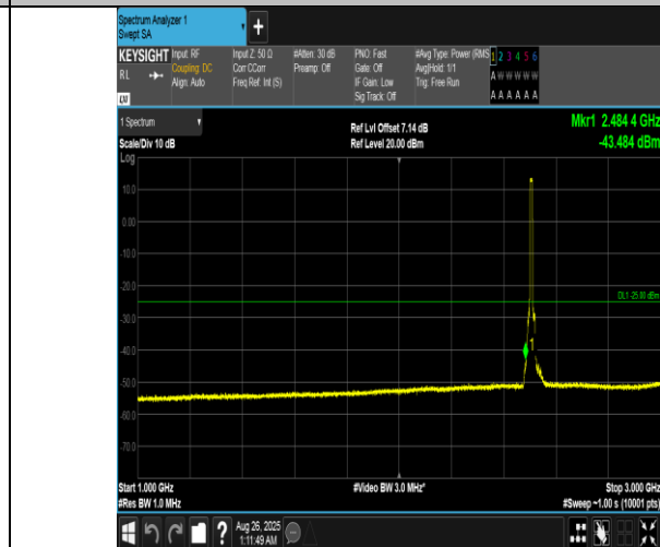
Band7-10MHz-QPSK-20800-50RB#0-1000~3000-PASS
