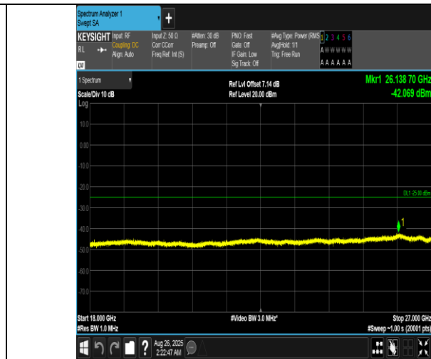
Band7-15MHz-QPSK-20825-1RB#74-18000~27000-PASS
