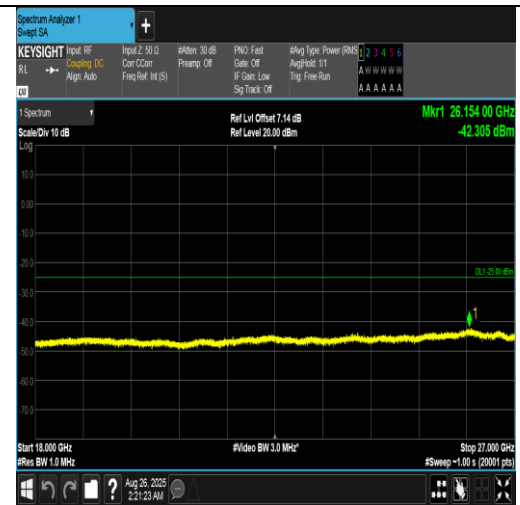
Band7-15MHz-16QAM-20825-1RB#0-18000~27000-PASS
