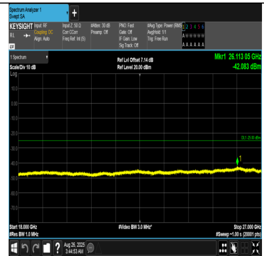
Band7-20MHz-QPSK-21100-1RB#99-18000~27000-PASS
