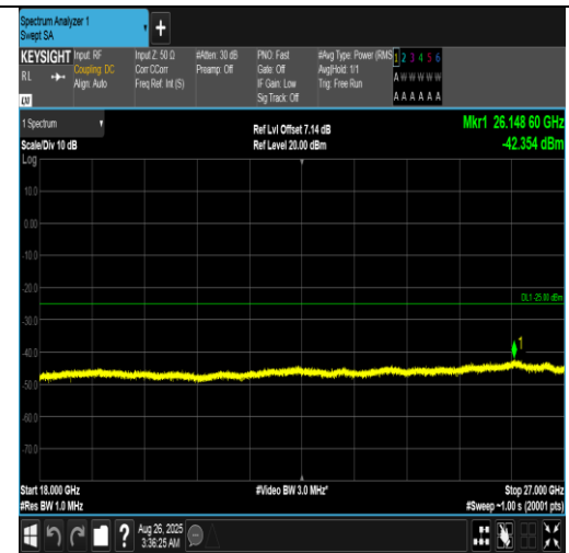
Band7-20MHz-QPSK-20850-1RB#99-18000~27000-PASS
