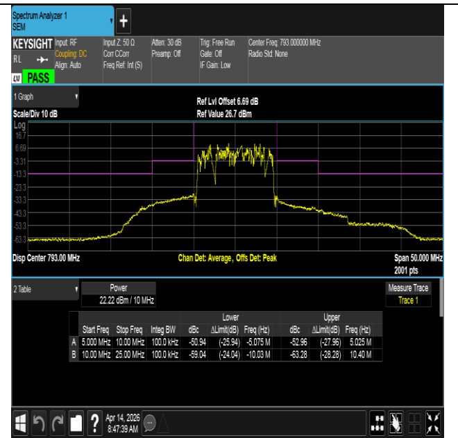
NTVN-Band14-10MHz-QPSK-23330-50RB#0--25.00--10.00-PASS
