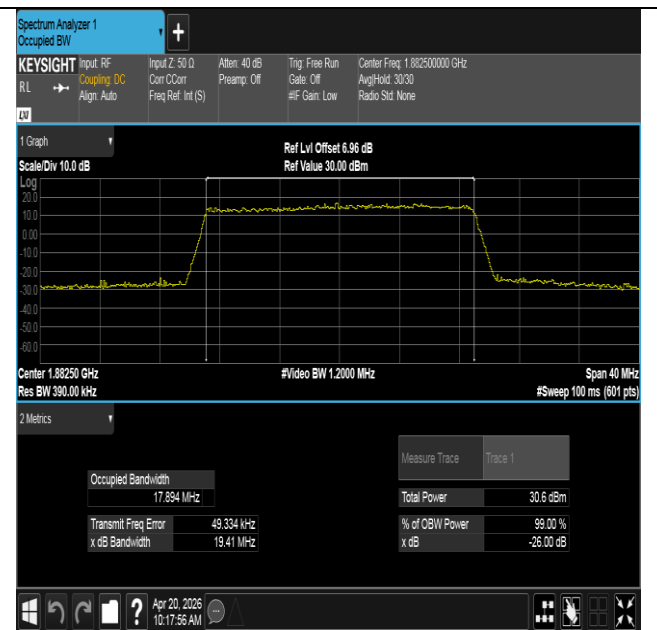
Band25-20MHz-16QAM-26365-100RB#0-PASS
