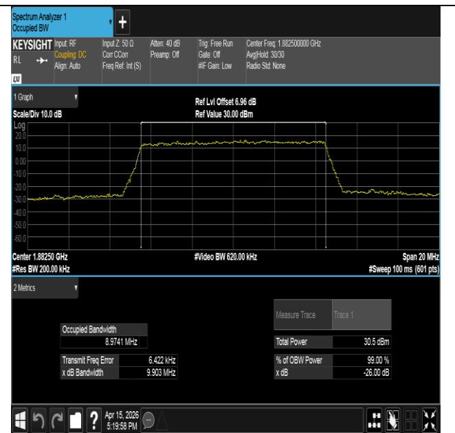
Band25-10MHz-16QAM-26365-50RB#0-PASS
