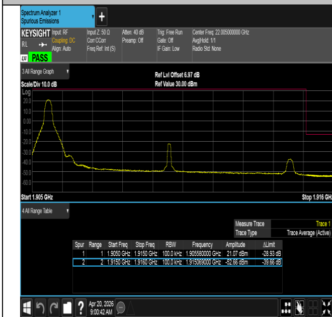
Band25-10MHz-QPSK-26640-1RB#0-PASS
