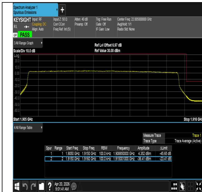
Band25-10MHz-QPSK-26640-50RB#0-PASS
