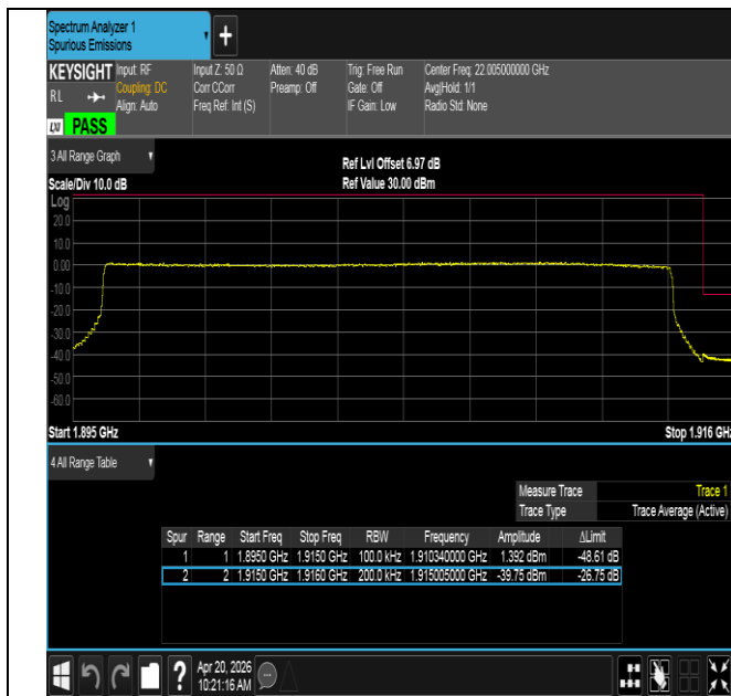
Band25-20MHz-QPSK-26590-100RB#0-PASS
