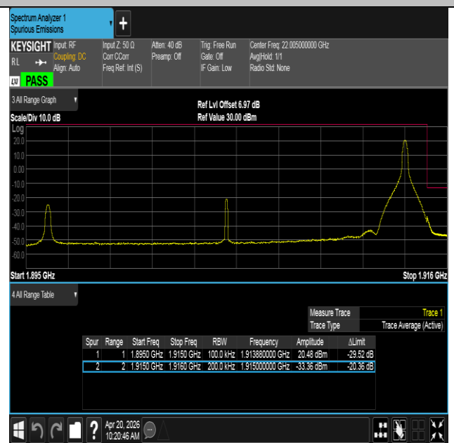
Band25-20MHz-QPSK-26590-1RB#99-PASS
