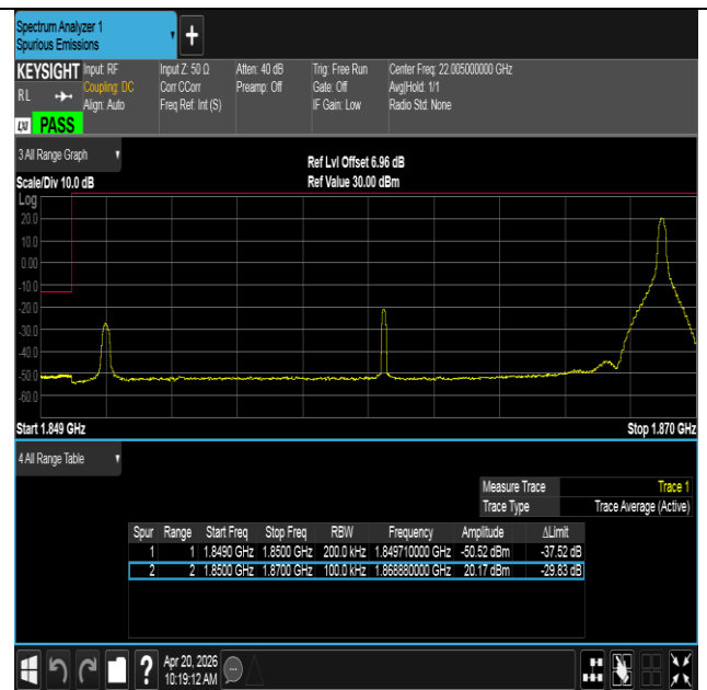
Band25-20MHz-QPSK-26140-1RB#99-PASS
