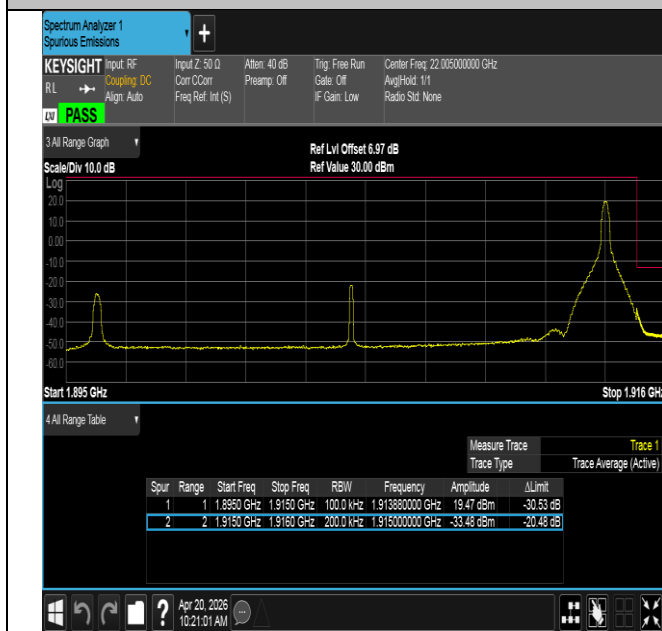
Band25-20MHz-16QAM-26590-1RB#99-PASS
