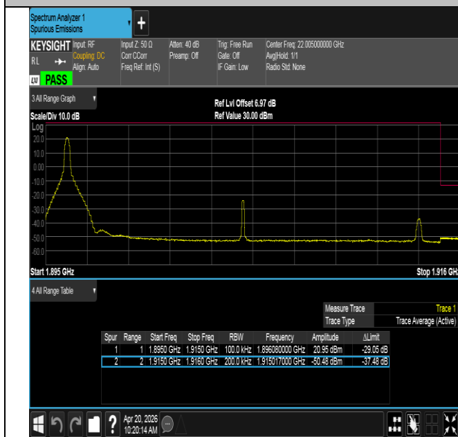
Band25-20MHz-QPSK-26590-1RB#0-PASS
