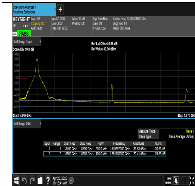
Band25-20MHz-QPSK-26140-1RB#0-PASS
