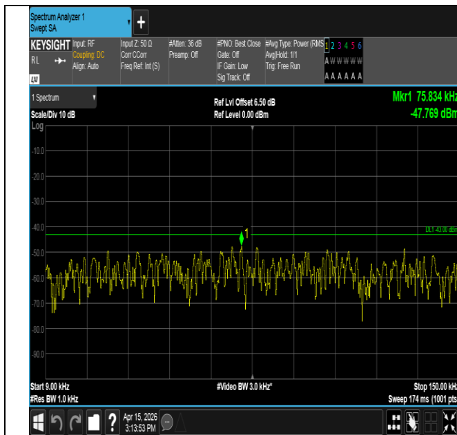
Band25-1.4MHz-QPSK-26365-6RB#0-0.009~0.15-PASS
