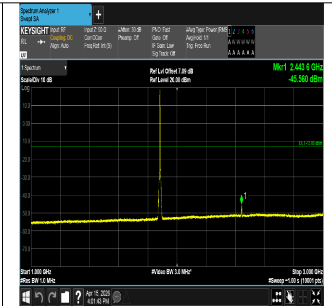
Band25-3MHz-QPSK-26365-15RB#0-1000~3000-PASS
