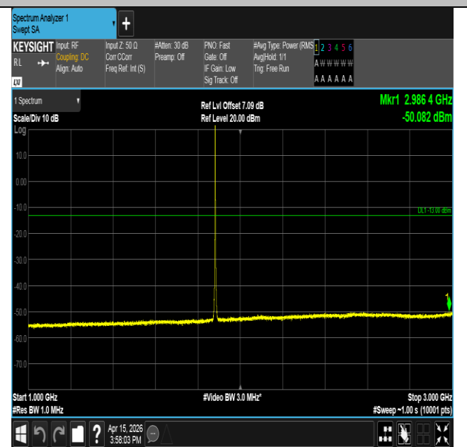
Band25-3MHz-QPSK-26365-1RB#0-1000~3000-PASS
