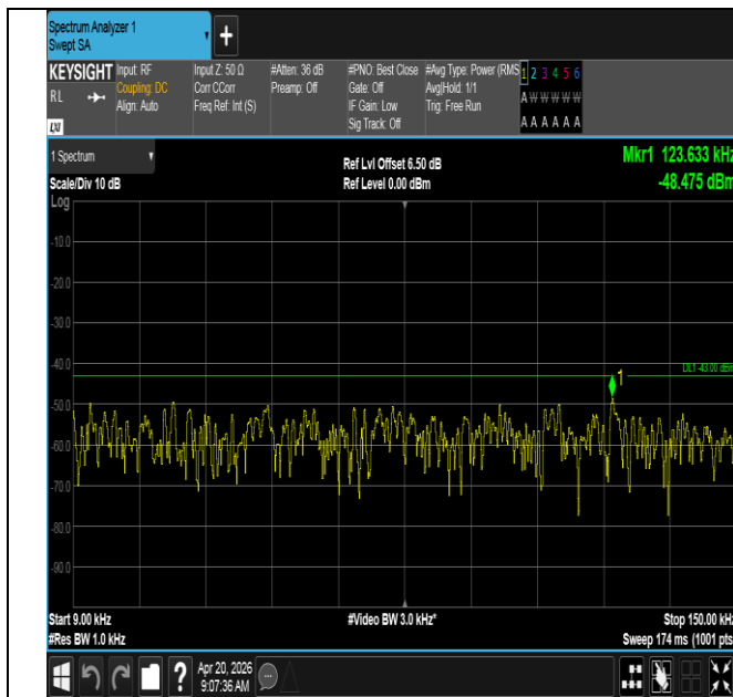
Band25-10MHz-QPSK-26365-1RB#0-0.009~0.15-PASS
