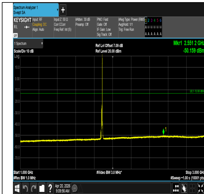
Band25-10MHz-QPSK-26365-1RB#49-1000~3000-PASS
