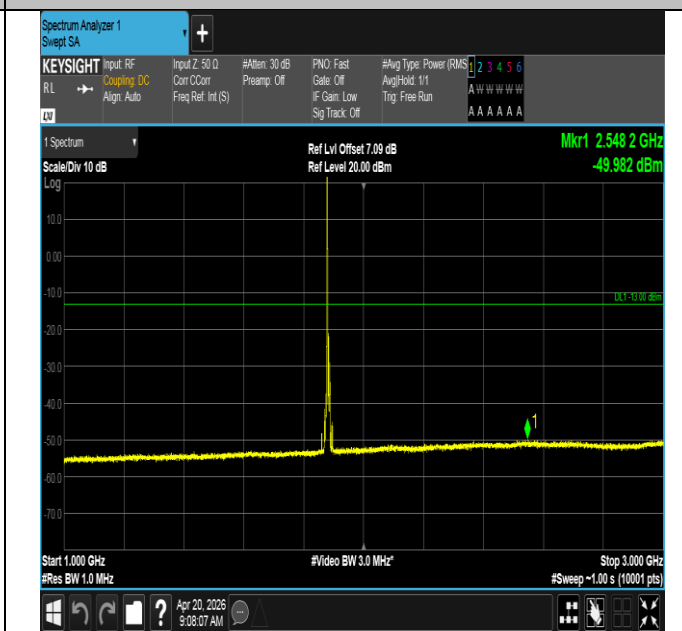
Band25-10MHz-QPSK-26365-1RB#0-1000~3000-PASS
