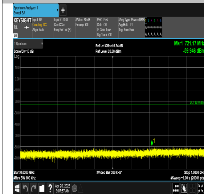
Band25-10MHz-QPSK-26365-1RB#0-30~1000-PASS
