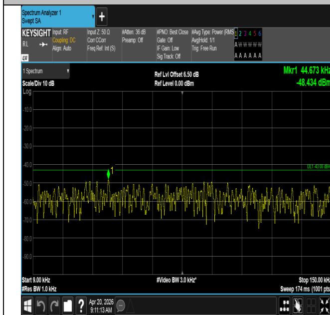
Band25-10MHz-QPSK-26365-50RB#0-0.009~0.15-PASS
