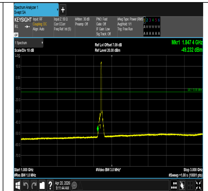
Band25-10MHz-QPSK-26365-50RB#0-1000~3000-PASS
