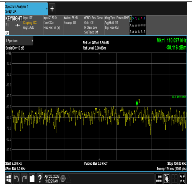
Band25-10MHz-QPSK-26365-1RB#49-0.009~0.15-PASS
