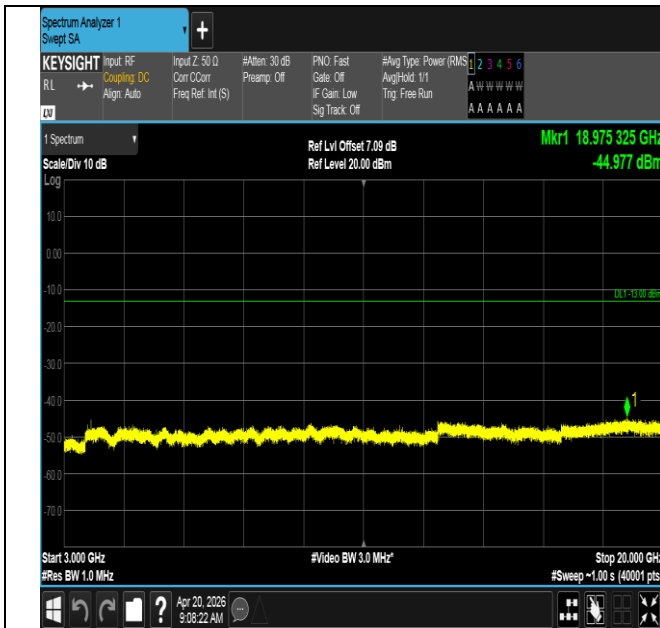
Band25-10MHz-QPSK-26365-1RB#0-3000~20000-PASS
