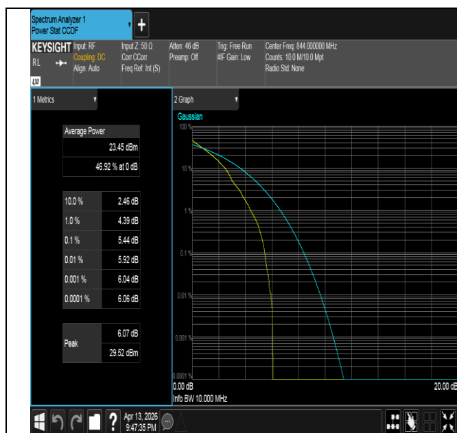
Band26(824-849)-10MHz-QPSK-26990-1RB#0-PASS
