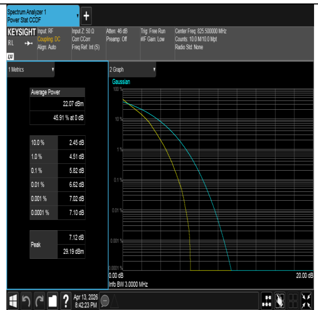
Band26(824-849)-3MHz-QPSK-26805-15RB#0-PASS
