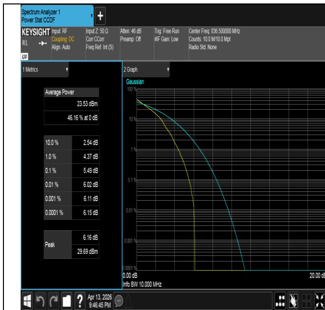
Band26(824-849)-10MHz-QPSK-26915-1RB#0-PASS
