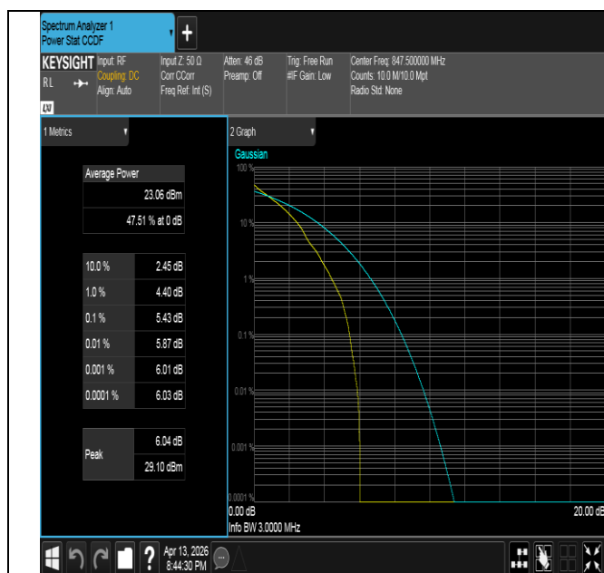
Band26(824-849)-3MHz-QPSK-27025-1RB#0-PASS
