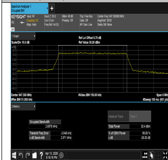
Band26(824-849)-3MHz-QPSK-27025-15RB#0-PASS
