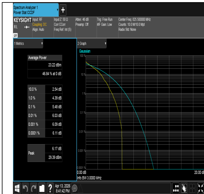
Band26(824-849)-3MHz-QPSK-26805-1RB#0-PASS
