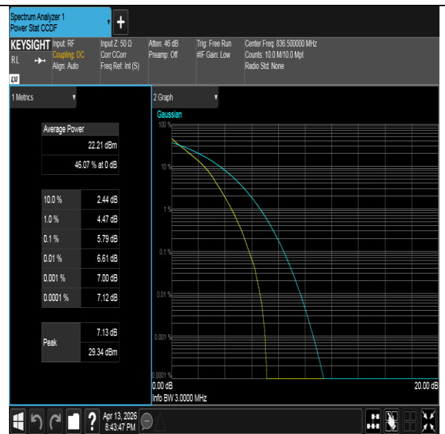
Band26(824-849)-3MHz-QPSK-26915-15RB#0-PASS
