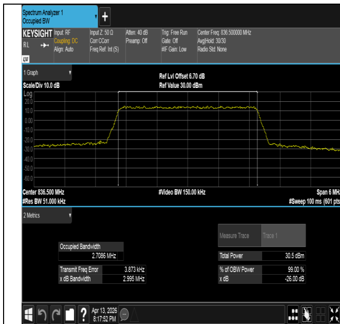
Band26(824-849)-3MHz-QPSK-26915-15RB#0-PASS
