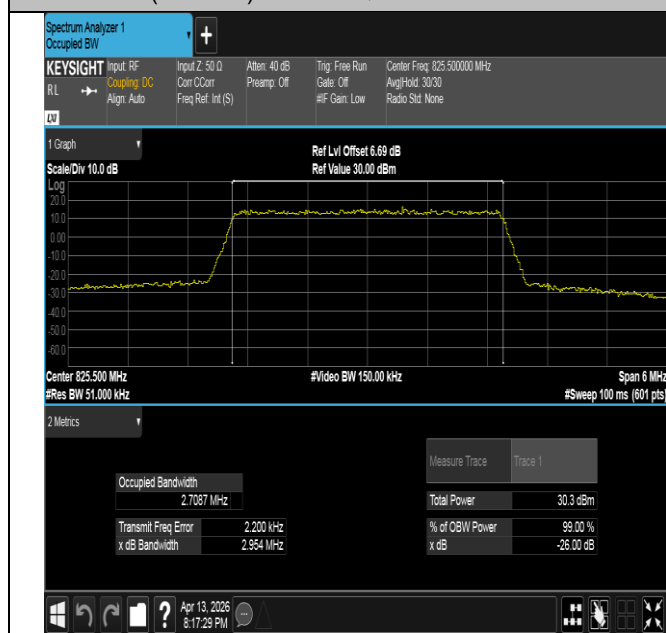
Band26(824-849)-3MHz-QPSK-26805-15RB#0-PASS
