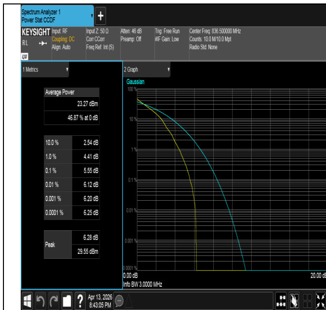
Band26(824-849)-3MHz-QPSK-26915-1RB#0-PASS
