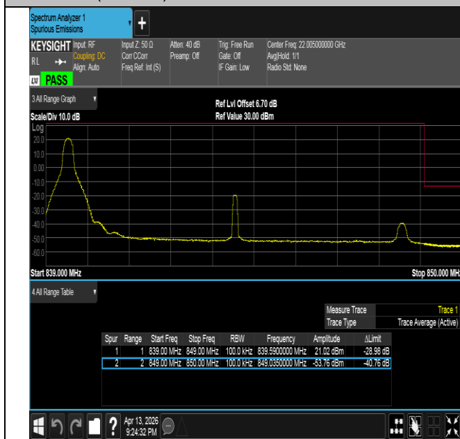
Band26(824-849)-10MHz-QPSK-26990-1RB#0-PASS
