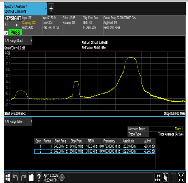
Band26(824-849)-3MHz-QPSK-27025-1RB#14-PASS
