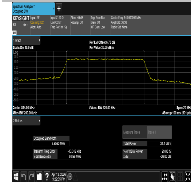
Band26(824-849)-10MHz-QPSK-26990-50RB#0-PASS
