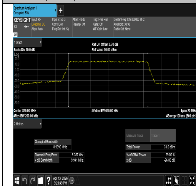
Band26(824-849)-10MHz-QPSK-26840-50RB#0-PASS
