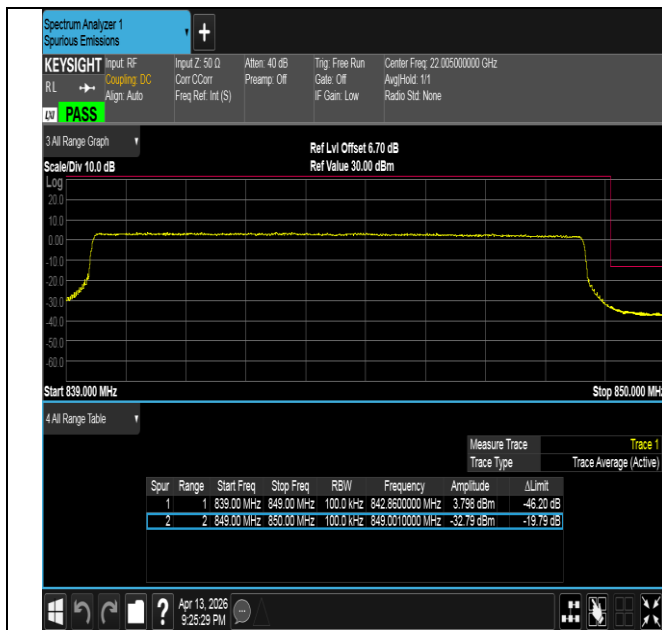
Band26(824-849)-10MHz-QPSK-26990-50RB#0-PASS
