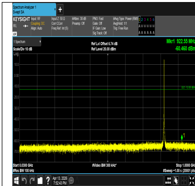
Band26(824-849)-1.4MHz-QPSK-26797-6RB#0-30~1000-PAS
