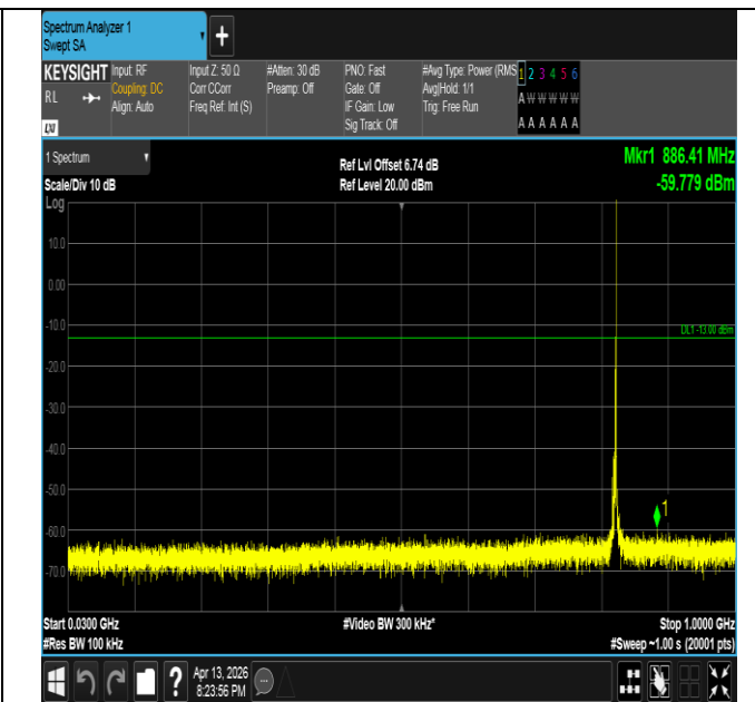
Band26(824-849)-3MHz-QPSK-26805-1RB#14-30~1000-PAS
