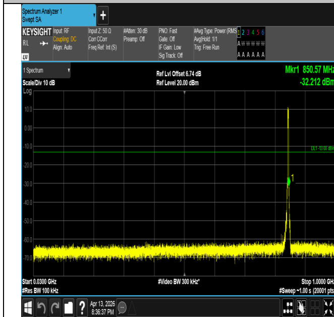
Band26(824-849)-3MHz-QPSK-27025-15RB#0-30~1000-PAS
