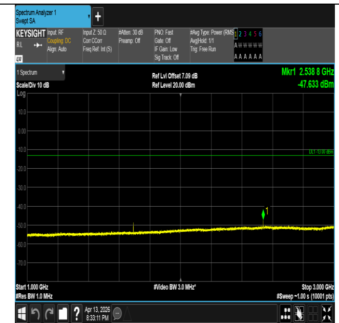
Band26(824-849)-3MHz-QPSK-27025-1RB#0-1000~3000-PASS SS
