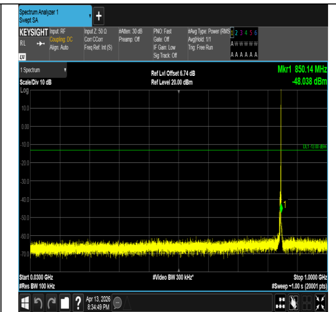
Band26(824-849)-3MHz-QPSK-27025-1RB#14-30~1000-PAS
