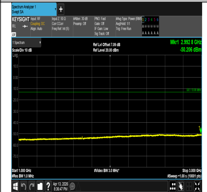
Band26(824-849)-3MHz-QPSK-27025-15RB#0-1000~3000-P
