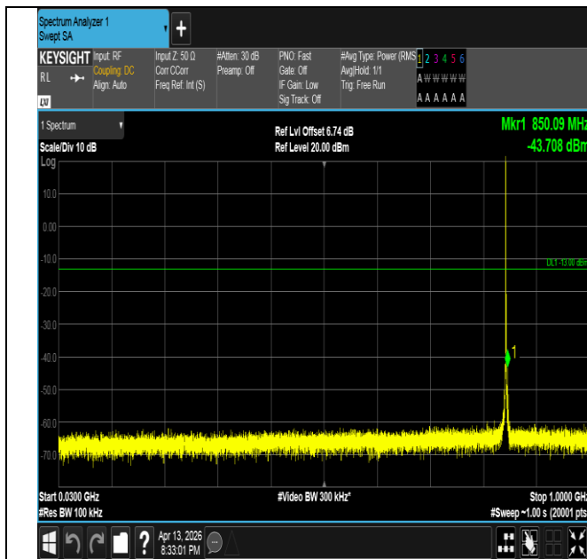
Band26(824-849)-3MHz-QPSK-27025-1RB#0-30~1000-PASS
