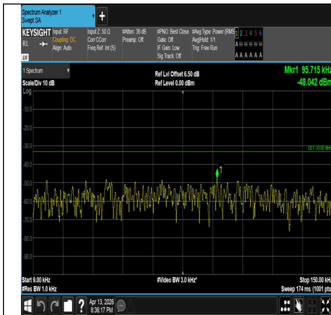
Band26(824-849)-3MHz-QPSK-27025-15RB#0-0.009~0.15-P
