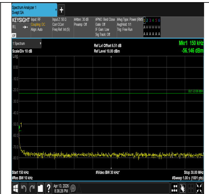
Band26(824-849)-3MHz-QPSK-27025-15RB#0-0.15~30-PAS
