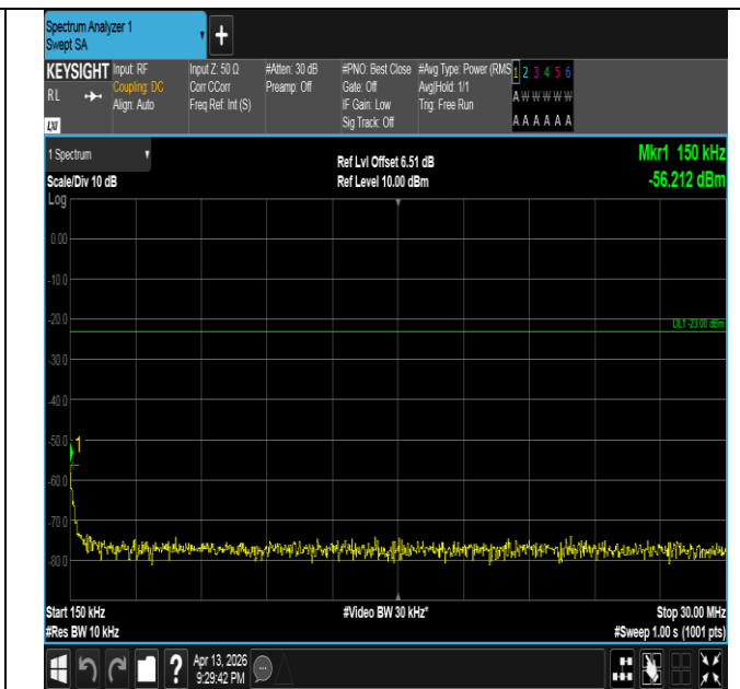
Band26(824-849)-10MHz-QPSK-26840-50RB#0-0.15~30-PAS S
