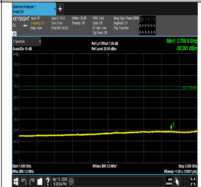
Band26(824-849)-10MHz-QPSK-26840-50RB#0-1000~3000-P ASS
