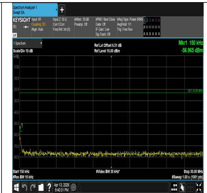
Band26(824-849)-10MHz-QPSK-26990-50RB#0-0.15~30-PAS S
