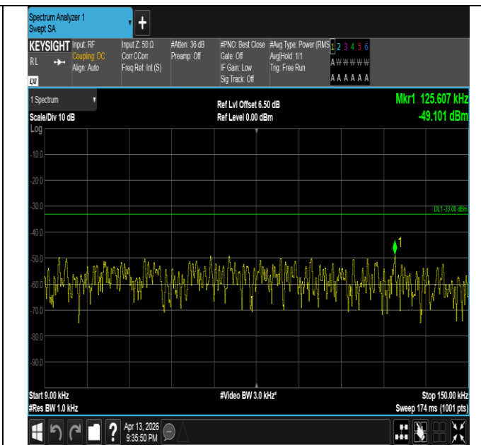
Band26(824-849)-10MHz-16QAM-26915-50RB#0-0.009~0.15 -PASS
