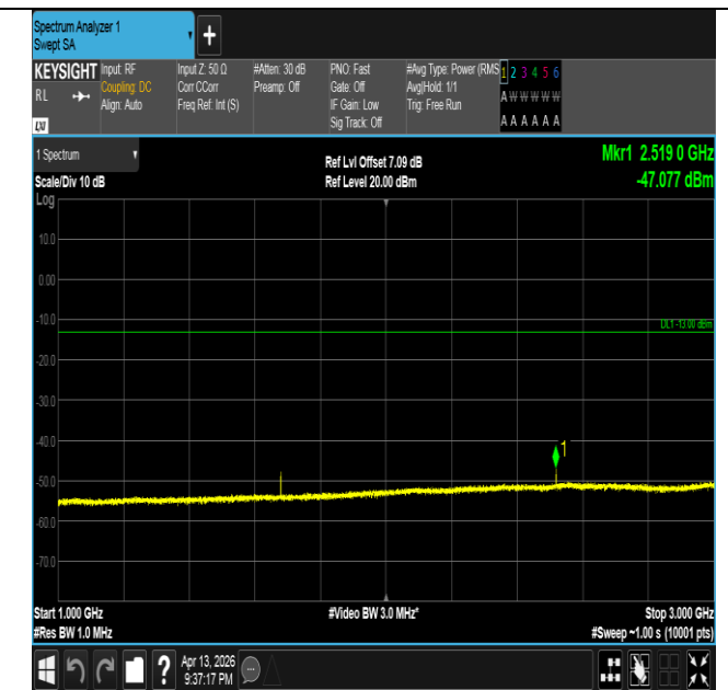
Band26(824-849)-10MHz-QPSK-26990-1RB#0-1000~3000-P
