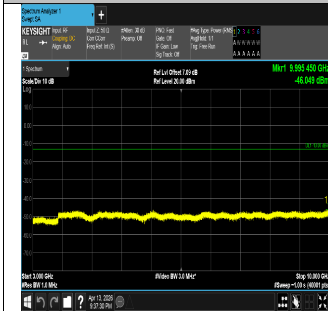
Band26(824-849)-10MHz-QPSK-26990-1RB#0-3000~10000-
