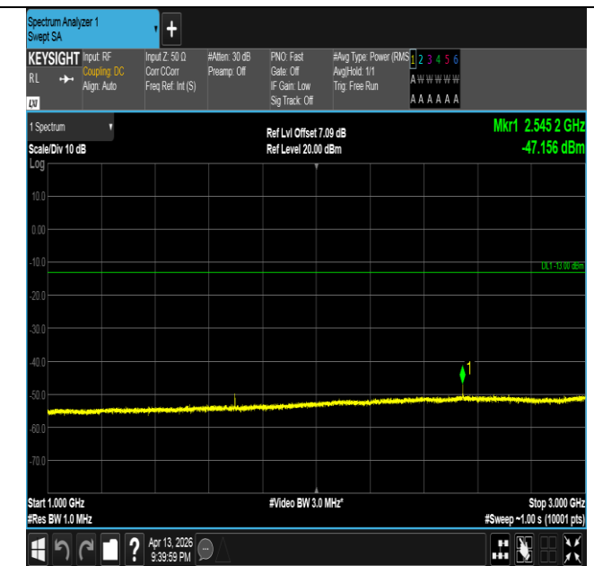
Band26(824-849)-10MHz-16QAM-26990-1RB#49-1000~3000 -PASS
