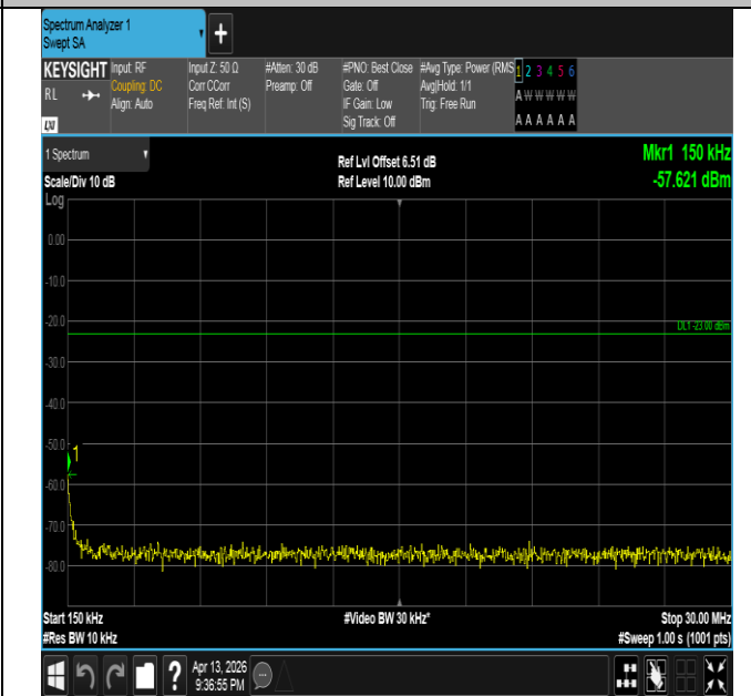
Band26(824-849)-10MHz-QPSK-26990-1RB#0-0.15~30-PAS
