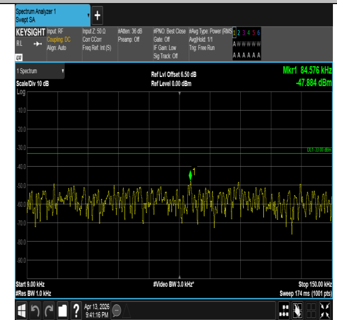
Band26(824-849)-10MHz-16QAM-26990-50RB#0-0.009~0.15 -PASS
