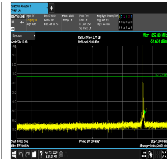
Band26(824-849)-10MHz-QPSK-26990-1RB#0-30~1000-PAS
