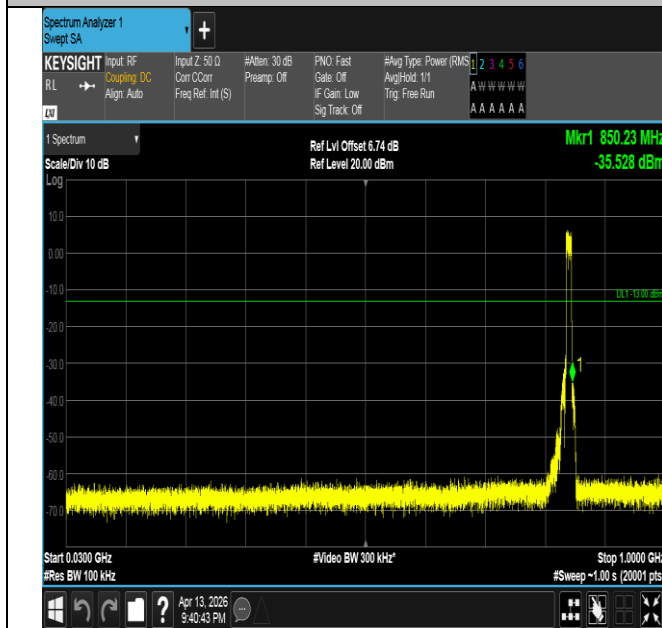
Band26(824-849)-10MHz-QPSK-26990-50RB#0-30~1000-PA SS
