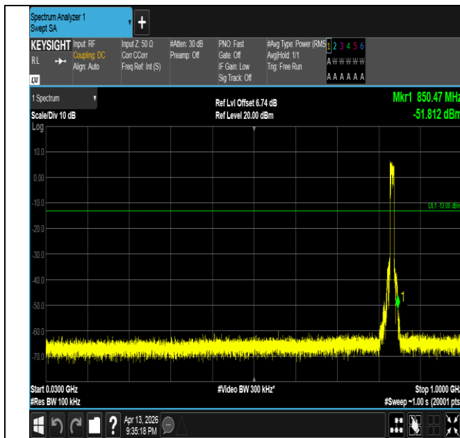
Band26(824-849)-10MHz-QPSK-26915-50RB#0-30~1000-PA SS
