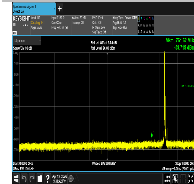
Band26(824-849)-10MHz-QPSK-26915-1RB#0-30~1000-PAS
