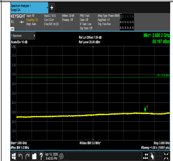
Band26(824-849)-10MHz-QPSK-26990-50RB#0-1000~3000-P ASS
