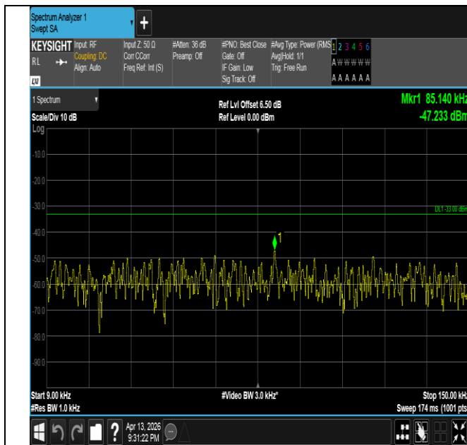
Band26(824-849)-10MHz-QPSK-26915-1RB#0-0.009~0.15-P
