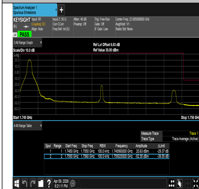
Band4-10MHz-QPSK-20350-1RB#0-PASS
