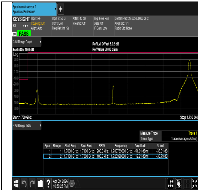
Band4-20MHz-16QAM-20050-1RB#99-PASS
