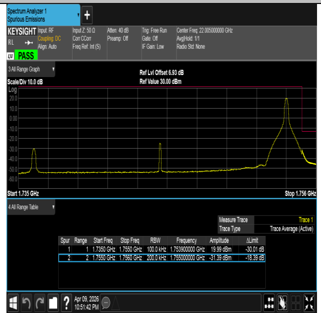
Band4-20MHz-QPSK-20300-1RB#99-PASS
