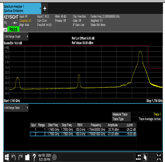
Band4-10MHz-QPSK-20350-1RB#49-PASS
