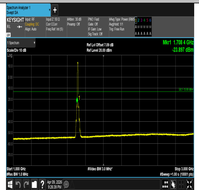
Band4-10MHz-QPSK-20000-50RB#0-1000~3000-PASS
