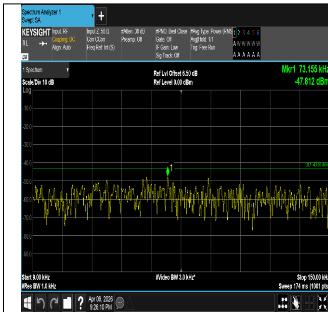
Band4-10MHz-QPSK-20000-50RB#0-0.009~0.15-PASS
