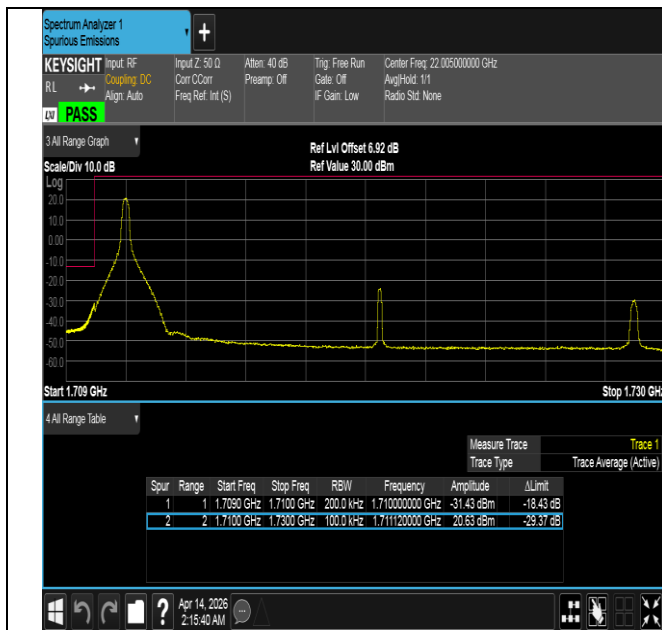
Band66-20MHz-QPSK-132072-1RB#0-PASS
