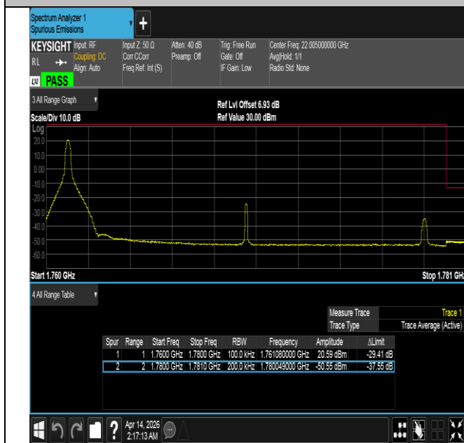
Band66-20MHz-QPSK-132572-1RB#0-PASS
