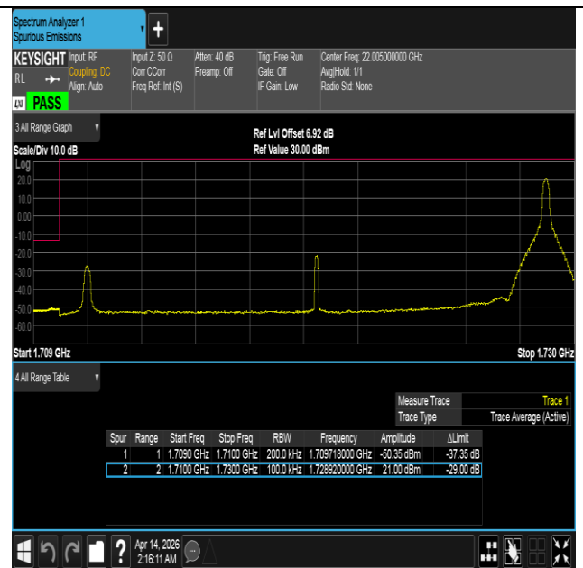
Band66-20MHz-QPSK-132072-1RB#99-PASS
