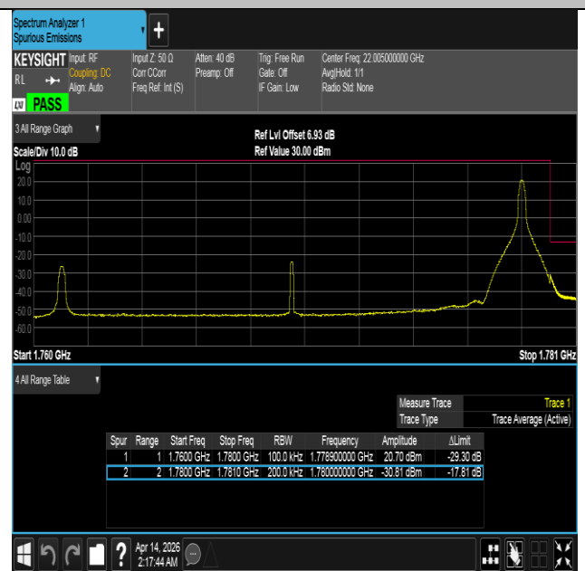
Band66-20MHz-QPSK-132572-1RB#99-PASS
