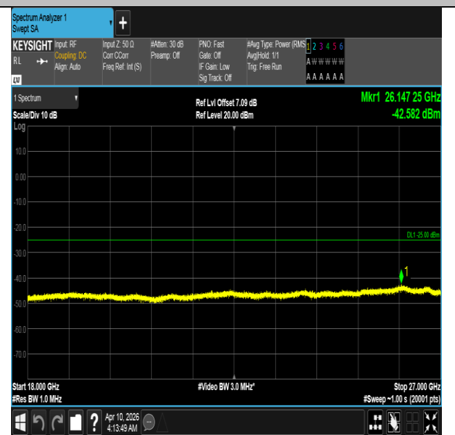
Band7-15MHz-QPSK-20825-1RB#0-18000~27000-PASS
