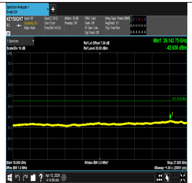
Band7-15MHz-16QAM-20825-1RB#0-18000~27000-PASS
