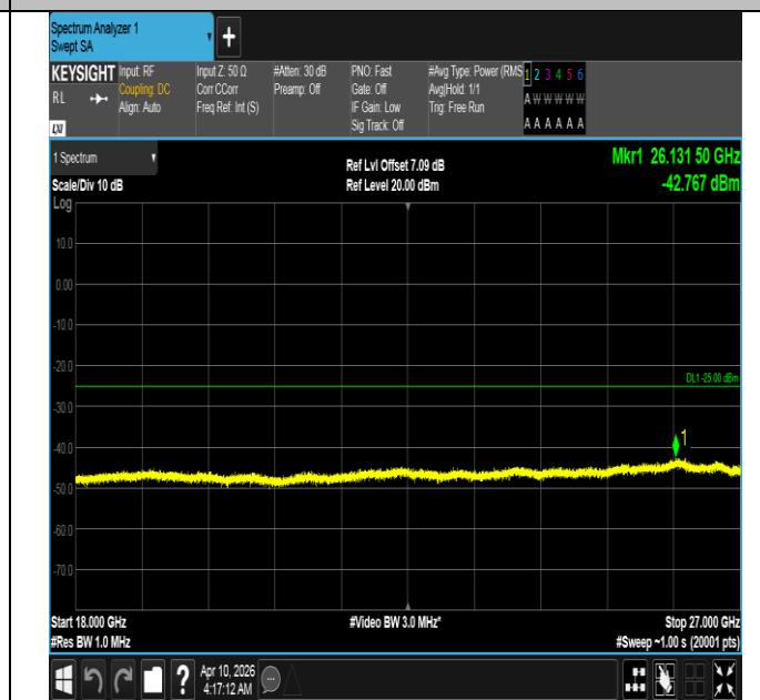
Band7-15MHz-16QAM-20825-1RB#74-18000~27000-PASS
