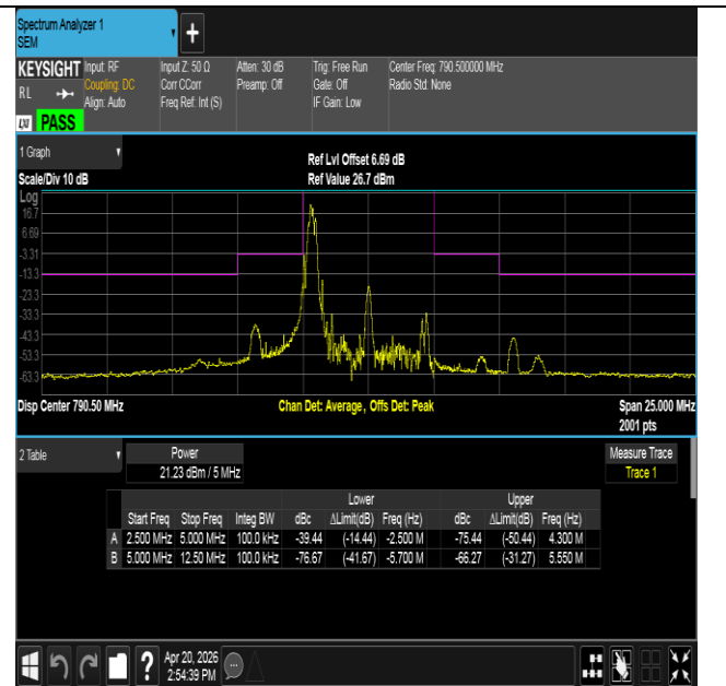
NTNV-Band14-5MHz-16QAM-23305-1RB#0--5.00--2.50-PAS
