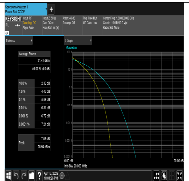
Band2-20MHz-QPSK-18900-100RB#0-PASS
