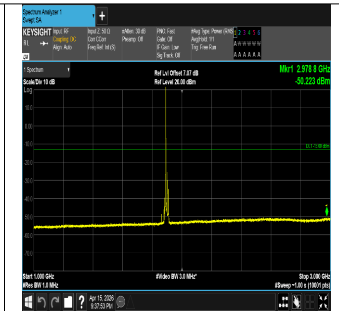
Band2-20MHz-QPSK-19100-1RB#0-1000~3000-PASS
