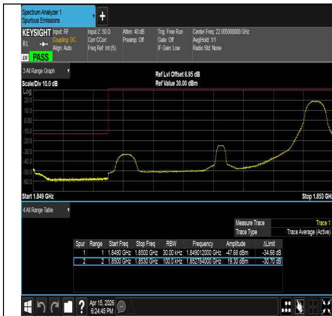
Band2-3MHz-16QAM-18615-1RB#14-PASS
