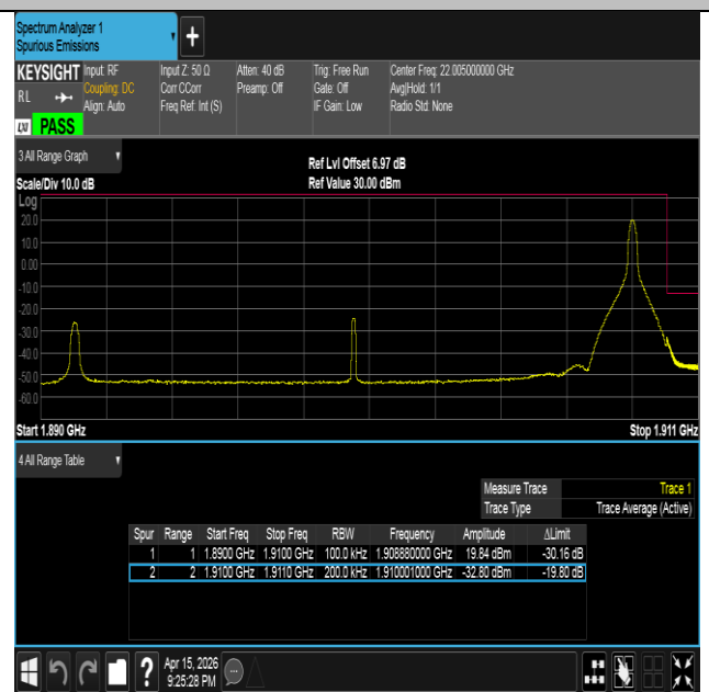
Band2-20MHz-QPSK-19100-1RB#99-PASS
