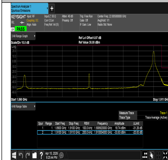
Band2-20MHz-16QAM-19100-1RB#99-PASS
