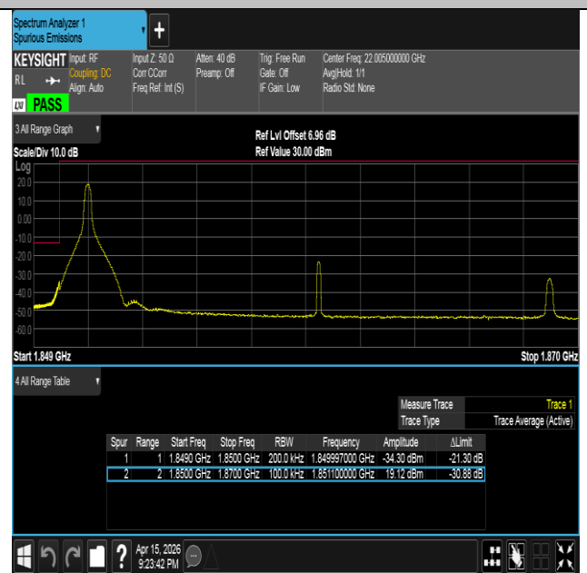
Band2-20MHz-16QAM-18700-1RB#0-PASS
