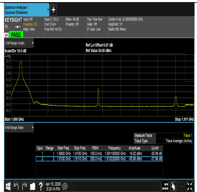
Band2-20MHz-16QAM-19100-1RB#0-PASS
