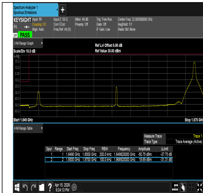
Band2-20MHz-16QAM-18700-1RB#99-PASS
