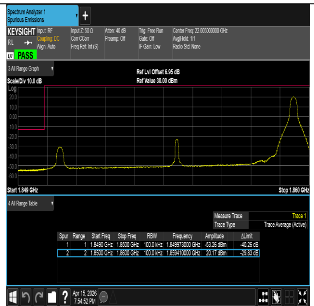
Band2-10MHz-QPSK-18650-1RB#49-PASS
