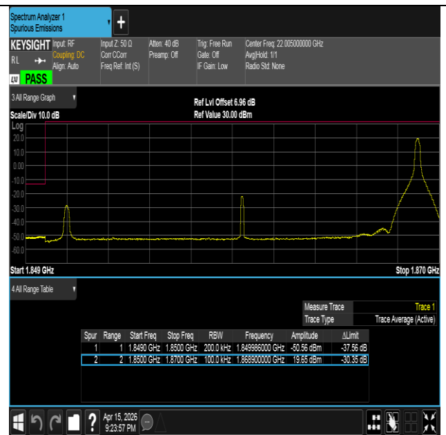
Band2-20MHz-QPSK-18700-1RB#99-PASS
