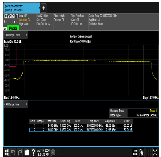
Band2-20MHz-16QAM-18700-100RB#0-PASS
