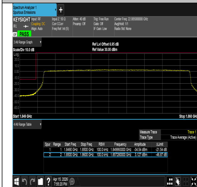
Band2-10MHz-QPSK-18650-50RB#0-PASS
