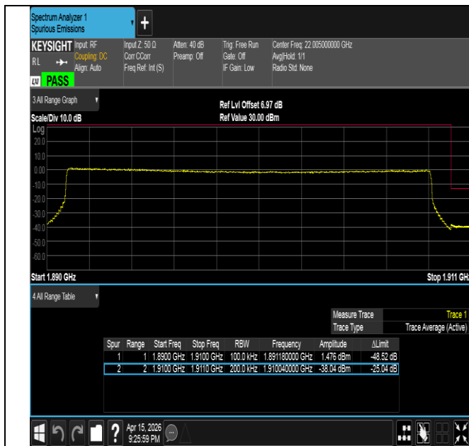
Band2-20MHz-QPSK-19100-100RB#0-PASS
