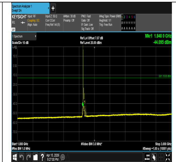
Band2-20MHz-QPSK-18700-1RB#0-1000~3000-PASS
