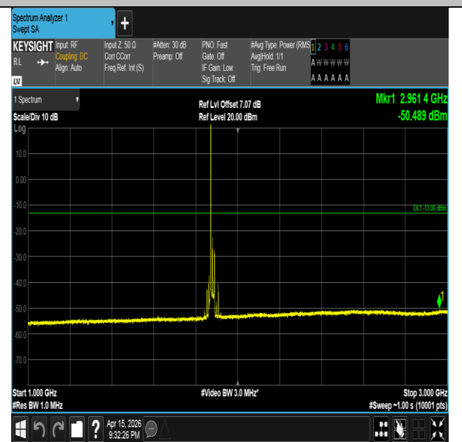
Band2-20MHz-QPSK-18900-1RB#0-1000~3000-PASS
