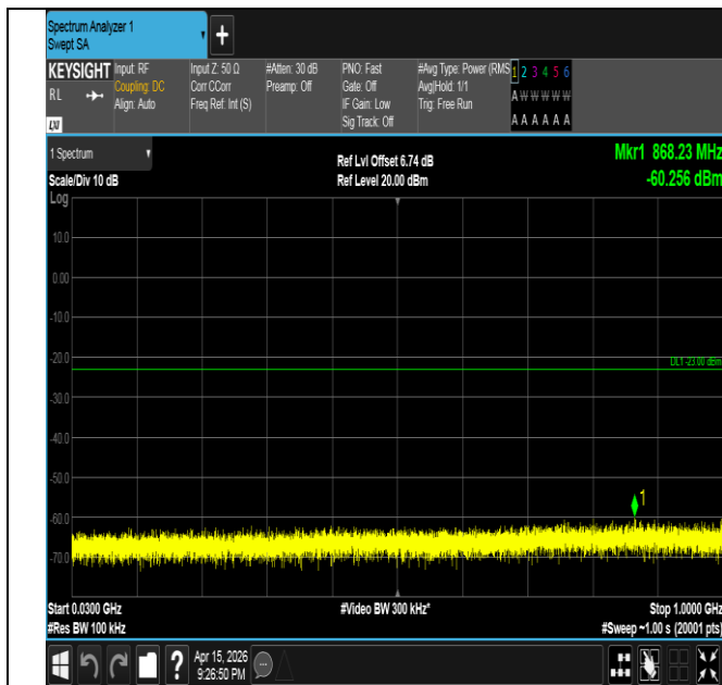
Band2-20MHz-QPSK-18700-1RB#0-30~1000-PASS
