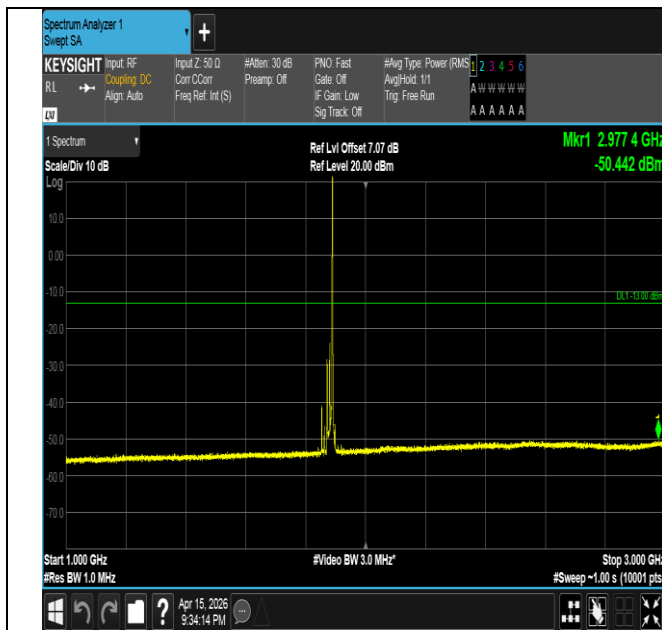
Band2-20MHz-QPSK-18900-1RB#99-1000~3000-PASS
